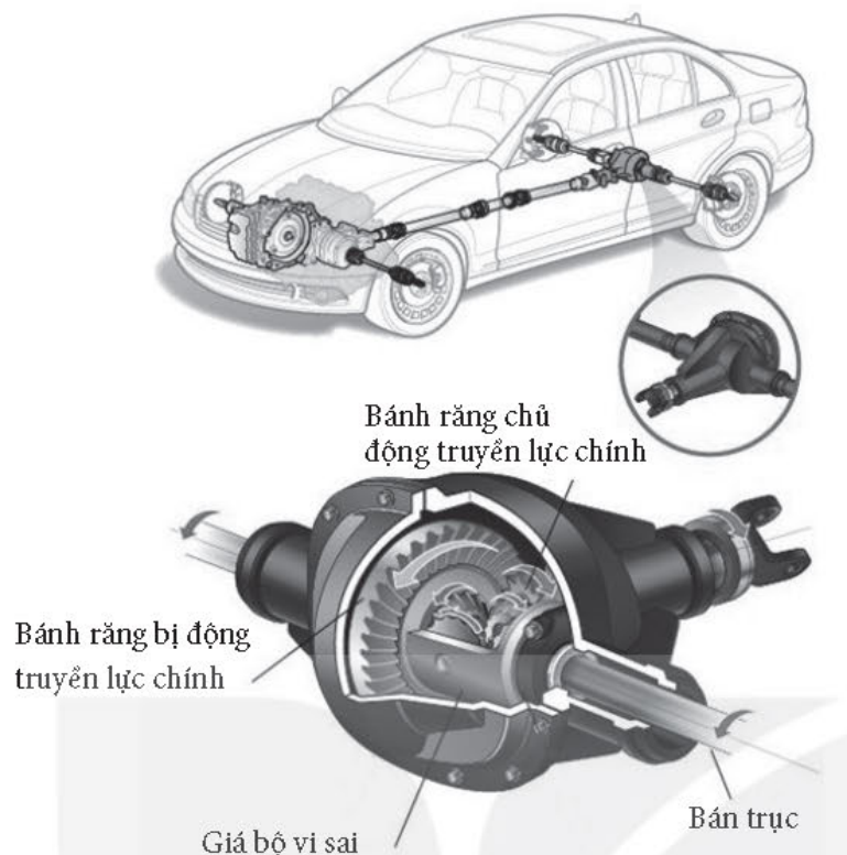
Hình 3. Vị trí của bộ truyền lực chính, vi sai trong hệ thống truyền lực và các bộ phận chính của chúng
