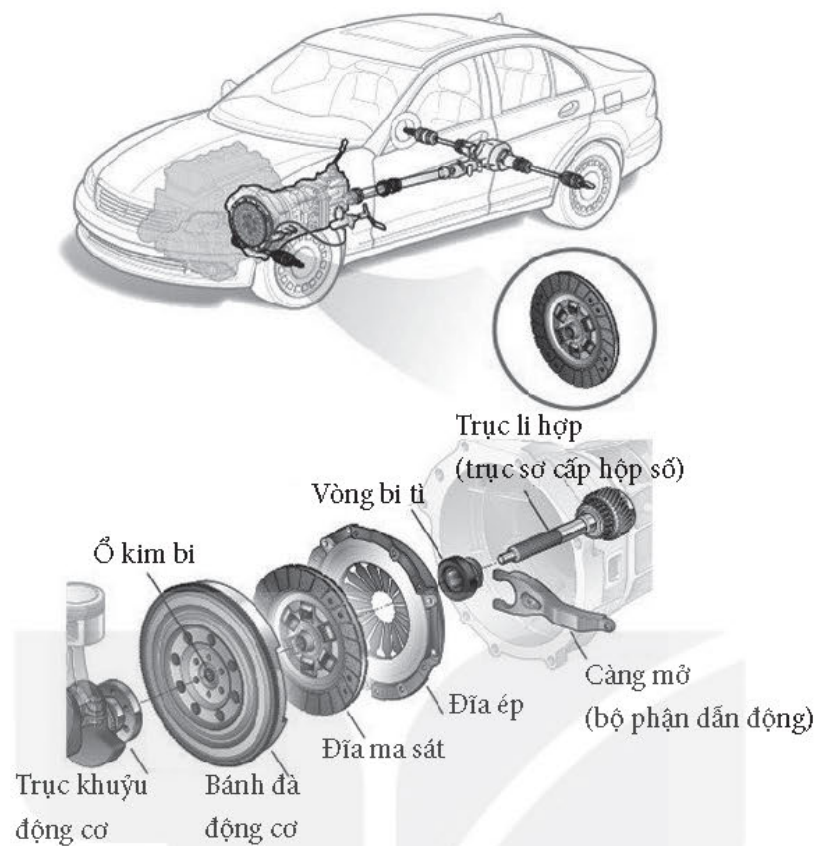
Hình 1. Vị trí của li hợp trong hệ thống truyền lực và các bộ phận chính của nó
