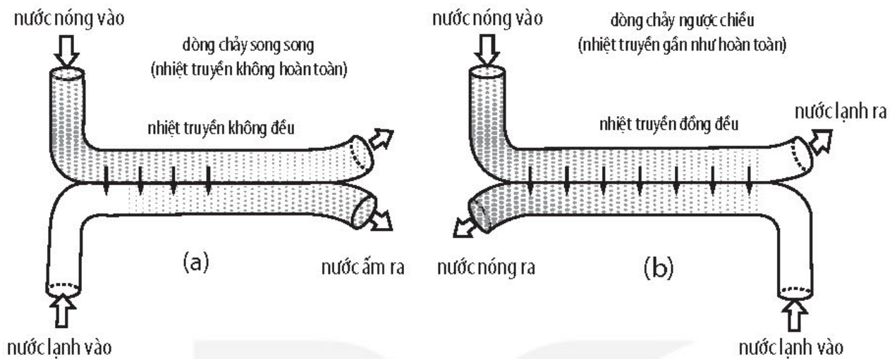
Hình 9.1. Trao đổi nhiệt giữa hai ống dẫn nhiệt tốt
