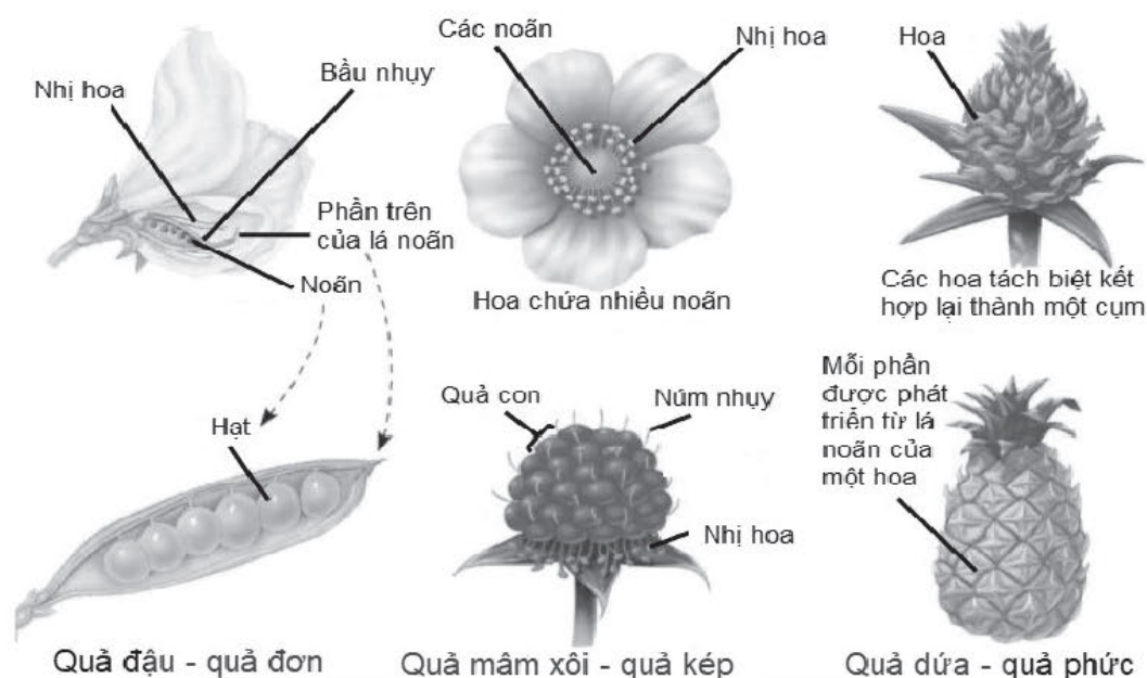
Hình 25.1. Các kiểu quả và nguồn gốc phát triển của chúng
