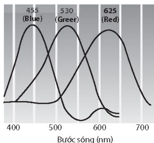
Hình 17.5. Ba bước sóng màu cơ bản
