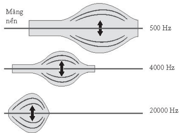
Hình 17.6. Màng nền dao động với tần số âm thanh từ thấp đến cao
