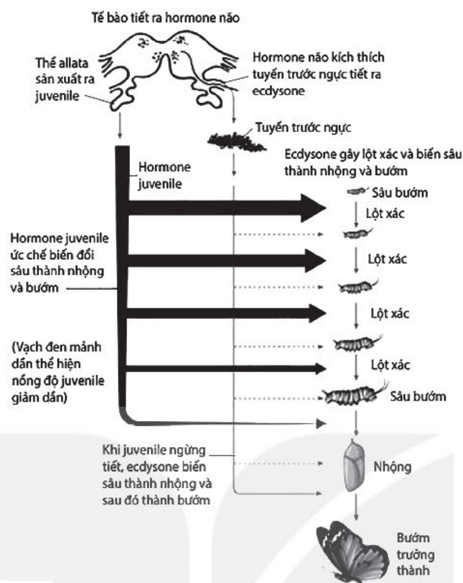
Hình 22.1. Tác động của hormone đến quá trình biến thái ở bướm
