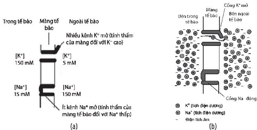
Hình 17.2. Phân bố K^+ và Na^+ hai bên màng tế bào và tính thấm của màng tế bào đối với K^+ và Na^+ (a), K^+ khuếch tán qua màng tế bào tạo ra phân cực ở hai bên màng (trong âm, ngoài dương) (b)
