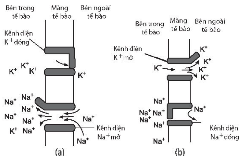
Hình 17.4. Di chuyển của các ion trong cơ chế hình thành điện thế hoạt động: giai đoạn khử cực và đảo cực (a) và giai đoạn tái phân cực (b)
