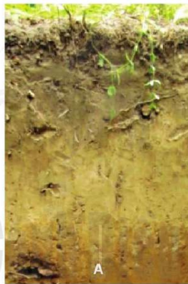
Hình 21.5. Mặt cắt thẳng đứng qua các tầng đất của đất pô-tôn (A) và đất pô-tôn có (B)
