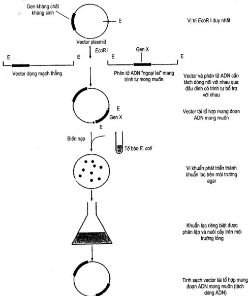
Hình 5.3. Tách dòng ADN bằng vector plasmid
