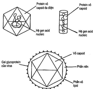
Hình 2.30. Cấu trúc virus lây nhiễm ở sinh vật nhân chuẩn. (a) dạng cấu trúc đa diện, (b) dạng sợi hoặc xoắn, (c) dạng có lớp vỏ lipid và gai glycoprotein
