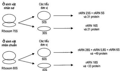
Hình 1.20. Thành phần cấu tạo điển hình của ribosom ở sinh vật nhân sơ (prokaryote) và sinh vật nhân chuẩn (eukaryote)
