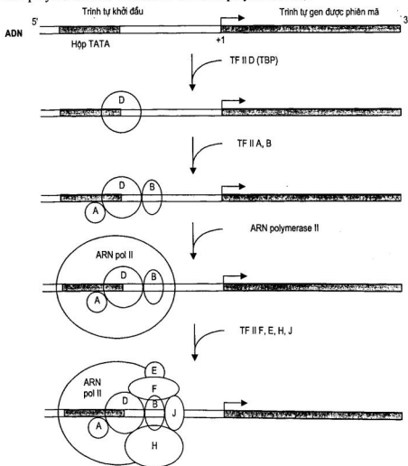
Hình 1.17. Quá trình gắn của enzyme ARN polymerase II và các yếu tố phiên mã vào trình tự khởi đầu phiên mã (promoter) ở sinh vật nhân chuẩn
