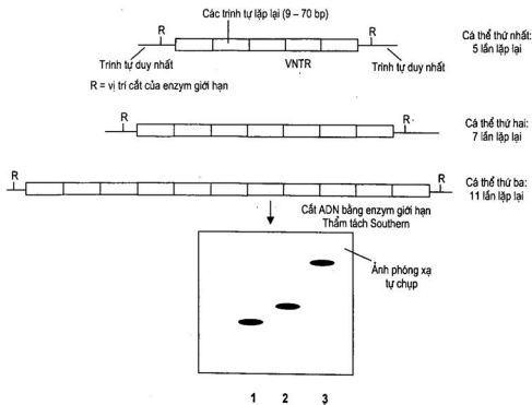
Hình 6.3. Chỉ thị đa hình VNTR có thể phát hiện được bằng kỹ thuật thẩm tách Southern và sử dụng để phân biệt các cá thể (sơ đồ trên đây minh họa ở cá thể đồng hợp tử).
