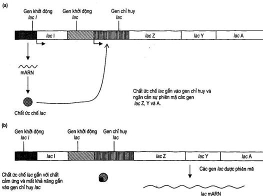
Hình 1.38. Sự điều hoà hoạt động của operon lac khi không có (a) và khi có chất cảm ứng (b)
