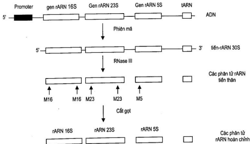
Hình 1.21. Quá trình phiên mã và hoàn thiện các ARN ribosom (rARN) ở E. coli
