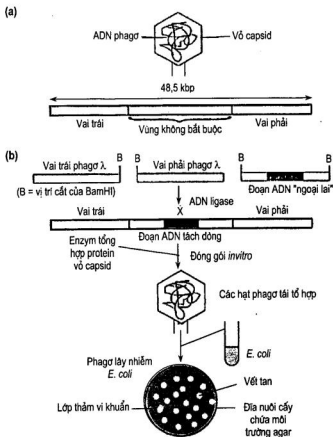
Hình 5.6. (a) Phagơ \lambda . (b) Sử dụng phagơ \lambda làm vector tách dòng
