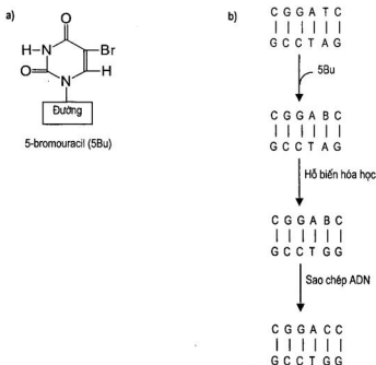
Hình 2.15. (a) Cấu trúc của 5-bromouracil; (b) Đột biến ADN gây ra bởi 5- bromouracil
