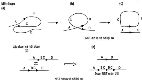
Hình 4.6. Mắt đoạn BC dưới dạng vòng tròn khép kín (a - c) có thể được tạo ra do đứt nối hoặc tái tổ hợp giữa các đoạn trình tự lặp lại trên cùng một NST, hoặc do các yếu tố di truyền vận động; vùng mắt đoạn/lập đoạn BC (d - e) có thể do đứt nối hoặc tái tổ hợp không theo hàng trên các NST tương đồng hoặc trên các nhiễm sắc tử chị em.
