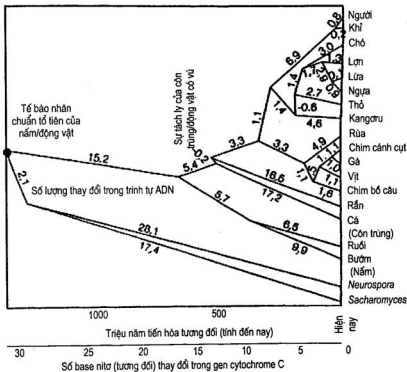
Hình 4.17. Cây tiến hoá (cây chủng loại phát sinh) của các loài động vật dựa trên sự thay đổi nucleotid trong gen cytochrome C. Các số liệu trên sơ đồ là số nucleotid trung bình thay đổi dọc theo mỗi nhánh. Nấm được sử dụng làm gốc của cây tiến hóa
