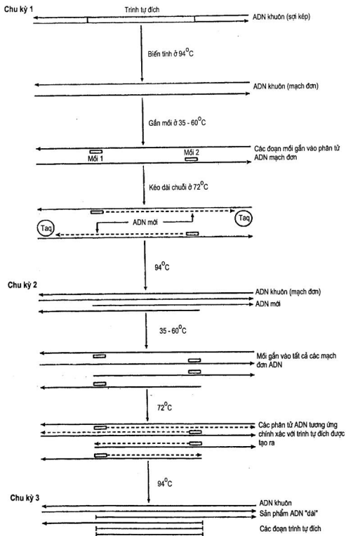
Hình 5.9. Phản ứng chuỗi trùng hợp - PCR
