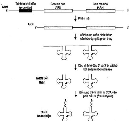
Hình 1.19. Quá trình phiên mã và hoàn thiện các phân tử tARN
