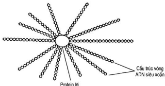
Hình 2.7. Cấu trúc nucleoid ở E. coli
