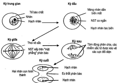
Hình 2.5. Sơ đồ quá trình nguyên phân ở tế bào động vật
