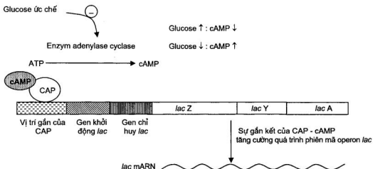
Hình 1.39. Ức chế operon lac bằng chất dị hoá
