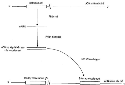
Hình 2.10 Sự vận động của yếu tố di truyền vận động kiểu phiên mã ngược (retroelement)
