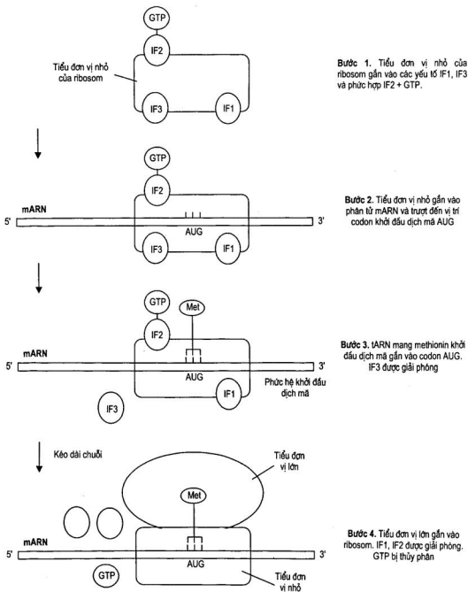
Hình 1.27. Sự khởi đầu dịch mã ở E. coli
