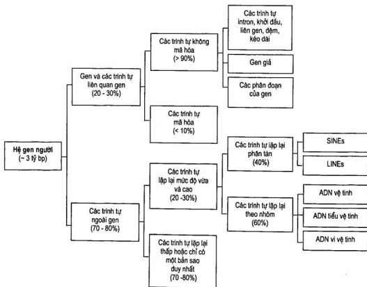
Hình 2.9. Các loại trình tự ADN trong hệ gen người
