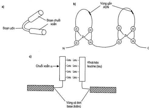
Hình 1.43. Các motif yếu tố phiên mã. (a) kiểu xoắn-uốn-xoắn, (b) kiểu ngón tay kẽm, và (c) Khóa kéo leucine và vùng gắn kết ADN có tính kiềm của yếu tố phiên mã Zip.
