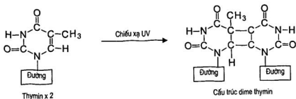
Hình 2.20. Sự hình thành cấu trúc thymine kép (dime thymine) do bức xạ UV
