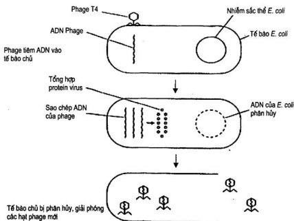
Hình 2.27. Sự nhiễm gây tan E. coli bởi phage T4
