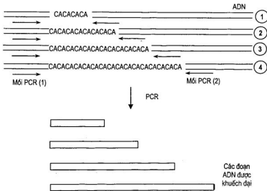
Hình 2.11. Các VNTR. Đoạn lặp [CA] lặp lại 4 - 16 lần. Kỹ thuật PCR dùng các đoạn mồi đặc hiệu đối với những trình tự nằm ở hai vùng biên của đoạn lặp để khuếch đại và tạo ra các đoạn ADN có độ dài khác nhau.
