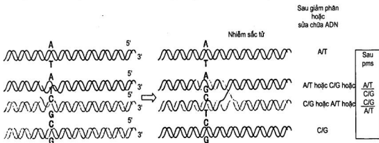
Hình 2.25. Sự biến trạng gen do sửa đổi ghép đôi sai ở chuỗi kép dị hợp ADN
