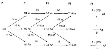
Hình 3.24. Mức độ gia tăng tính đồng hợp tử qua các thế hệ liên tục tự thụ phấn (sự nội phối cực đoan)
