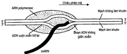
Hình 1.15. Giai đoạn kéo dài phiên mã
