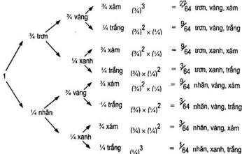
Hình 3.28. Xác suất tần số kiểu hình ở F2 trong một phép lai ba tính theo nguyên tắc di truyền học Mendel được tính theo nguyên tắc nhân xác suất
