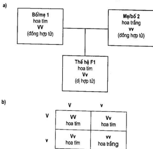
Hình 3.1. (a) Các giao tử do cây F1 sinh ra mang alen V hoặc v kết hợp ngẫu nhiên, tạo ra thế hệ con có các kiểu gen VV , Vv , vv như được thể hiện ở (b). (b) Mỗi trong số bốn kiểu kết hợp giao tử xuất hiện với tần số bằng nhau. Vì vậy tần số kiểu hình ở F2 là 3 tím : 1 trắng và tần số kiểu gen là 1 VV : 2 Vv : 1 vv .
