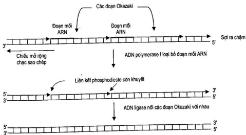
Hình 1.34. Hoàn thành tổng hợp sợi ra chậm (sợi theo sau)
