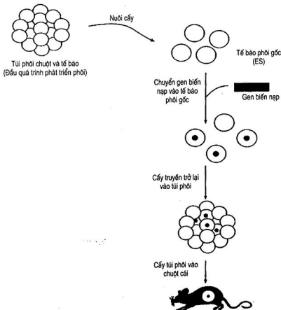
Hình 6.18. Chuyển gen ở động vật thông qua tế bào phôi gốc (ES)
