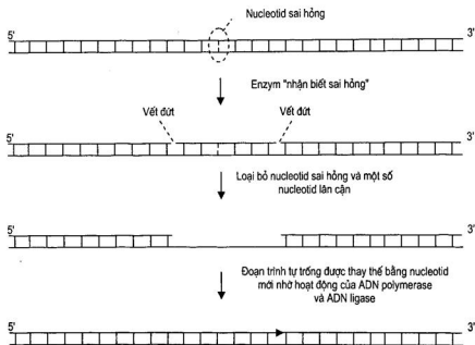
Hình 2.21. Sửa chữa ADN bằng cắt bỏ
