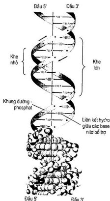
Hình 1.5. Chuỗi xoắn kép ADN
