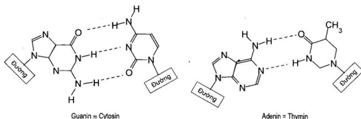
Hình 1.6. Các cặp base nitơ liên kết bổ trợ (liên kết hydro được minh họa bằng vạch ngắt quãng)
