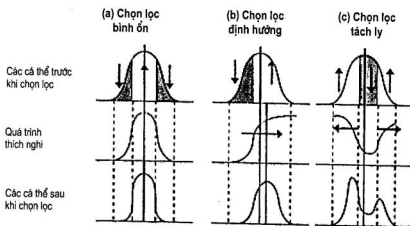
Hình 4.1. Các phương thức chọn lọc. Vùng đậm là vùng bị chọn lọc đào thải. Những mũi tên chỉ hướng biến đổi tần số kiểu hình theo thời gian. Đường liền, thẳng đứng là giá trị trung bình, các đường gạch nối để so sánh.
