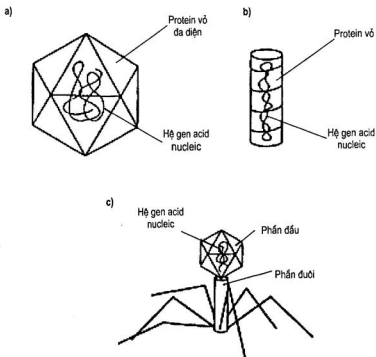
Hình 2.26. Cấu trúc của phage. (a) dạng đa diện, (b) dạng sợi hoặc xoắn, (c) dạng có cấu trúc đầu và đuôi
