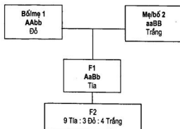
Hình 3.6. Tỷ lệ phân ly 9 : 7
