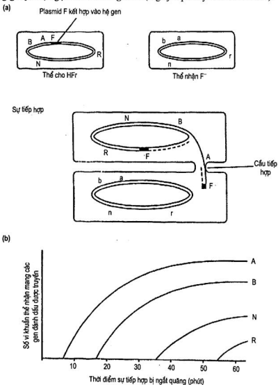
Hình 3.15. (a) Vi khuẩn thể cho HFr và vi khuẩn thể nhận F. HFr mang plasmid F được lồng ghép vào NST của nó. Bốn gen đánh dấu A, B, N và R để chọn lọc được thể hiện ở các vị trí tương ứng trên bản đồ gen. Thể nhận mang các gen lặn của bốn gen đó (ký hiệu bằng chữ thường). Trong quá trình tiếp hợp, NST bị gãy bên trong yếu tố F. Sợi đơn ADN được truyền qua ống tiếp hợp. Chú ý rằng, sợi này được sao chép bên trong thể nhận và quá trình tổng hợp sợi mới thứ hai cũng được bắt đầu ở thể cho ở vùng cách xa yếu tố F, được biểu diễn bằng đường chấm. Đó là sự sao chép vòng lặp. (b) Trật tự và vị trí của các gen A, B, N và R được xác định bằng cách lập đồ thị số lượng vi khuẩn nhận mang các dấu chuẩn chọn lọc tại các thời điểm khác nhau khi sự tiếp hợp bị ngắt quãng. Đồ thị cho thấy vị trí tương đối của các gen đánh dấu là: A – 8 phút; B – 17 phút; N – 36 phút; R – 54 phút kể từ điểm khởi đầu truyền gen.
