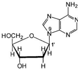
a) 2'-deoxyadenosin (nucleozid)
