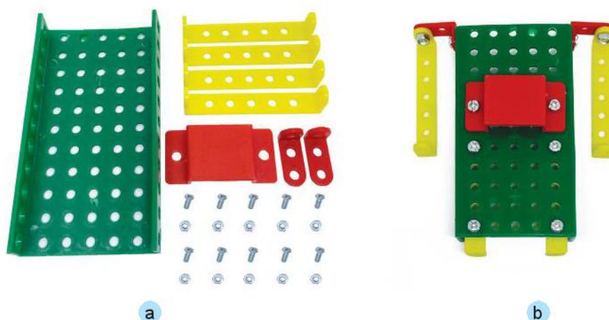
Hình 3 Các chi tiết và thân rô-bốt
