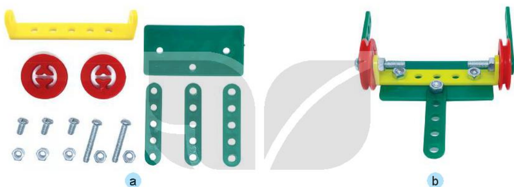
Hình 2 Các chi tiết và đầu rô-bốt
