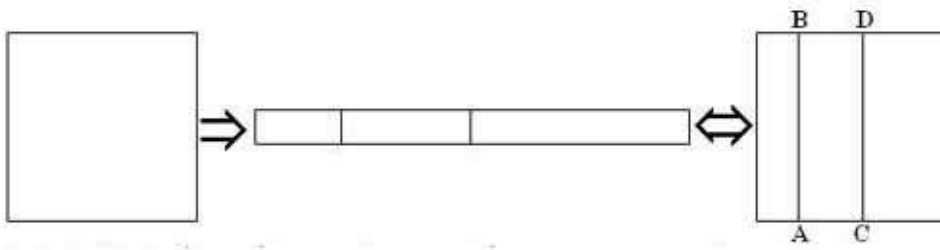
Hình 17: Ép và cắt, tương đương việc cắt các đường song song với cạnh tam giác.
