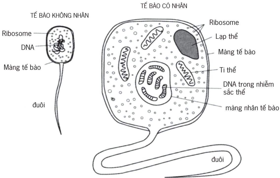
Hình 2.2 So sánh tế bào có nhân và tế bào không nhân
