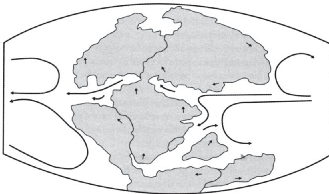
Hình 2.3 Sự phân tách của Pangaea khoảng 200 triệu năm trước
