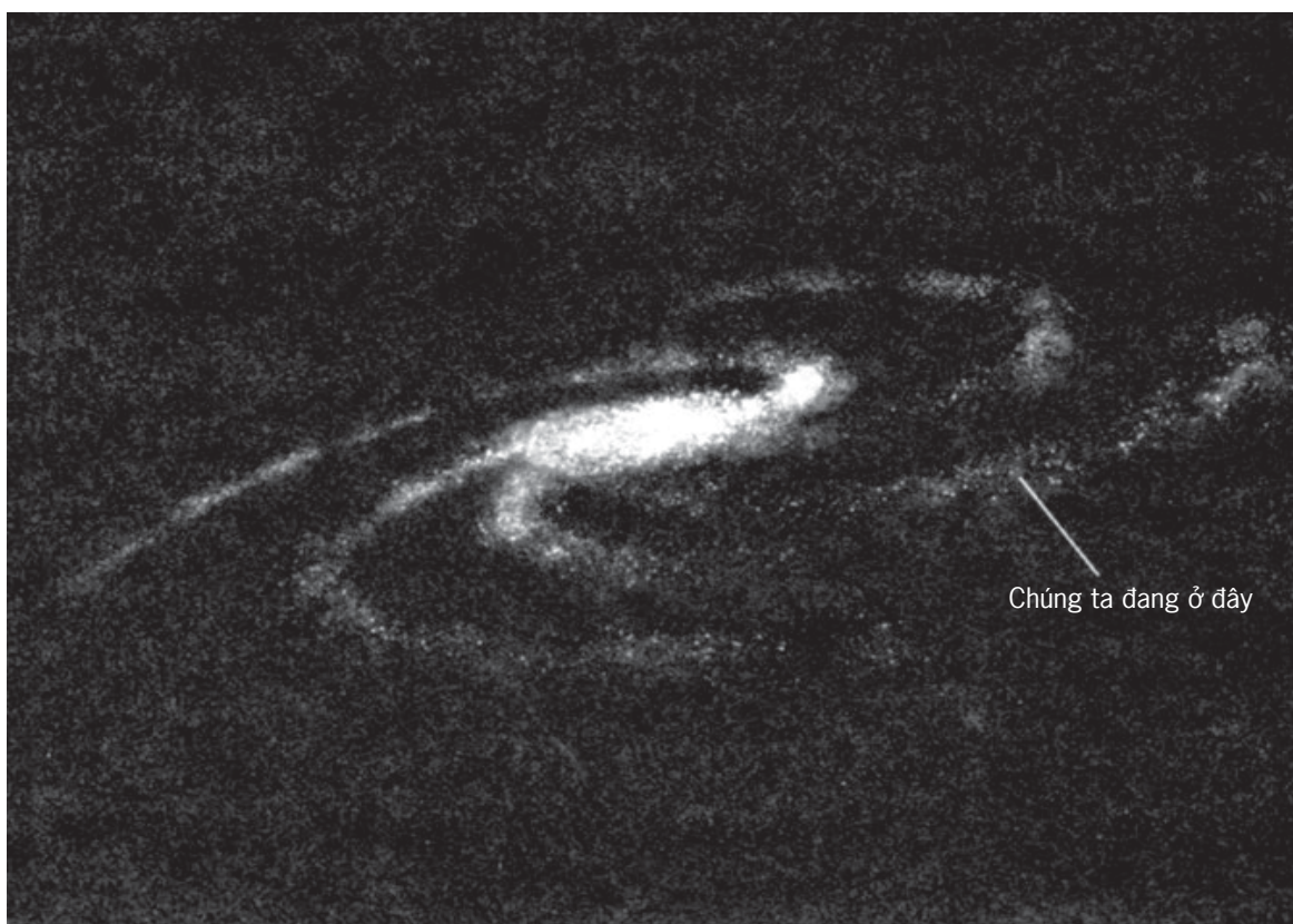
Hình 1.1 Ngân hà
