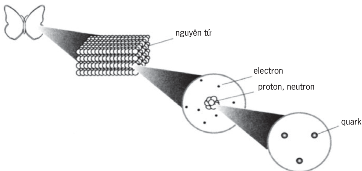
Hình 1.2 Thành phần của vật chất
