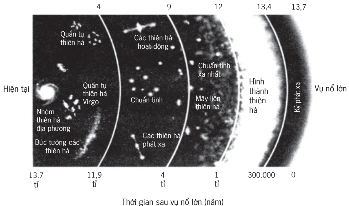
Hình 1.3 Vũ trụ như chúng ta thấy
