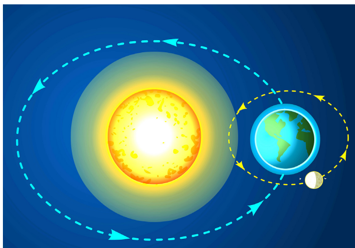
▲ Hình 25.1. Trái đất quay quanh Mặt Trời
