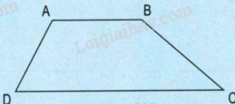
Hình thang ABCD
