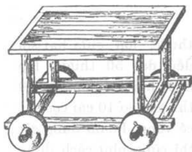
Hình 38. Xe trâu gỗ dây mà kéo. Phàm đánh thành muốn leo lên thì lấy màn gỗ che trước mặt cho khỏi tên đạn.
