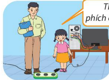
Hình 17. An toàn về điện
