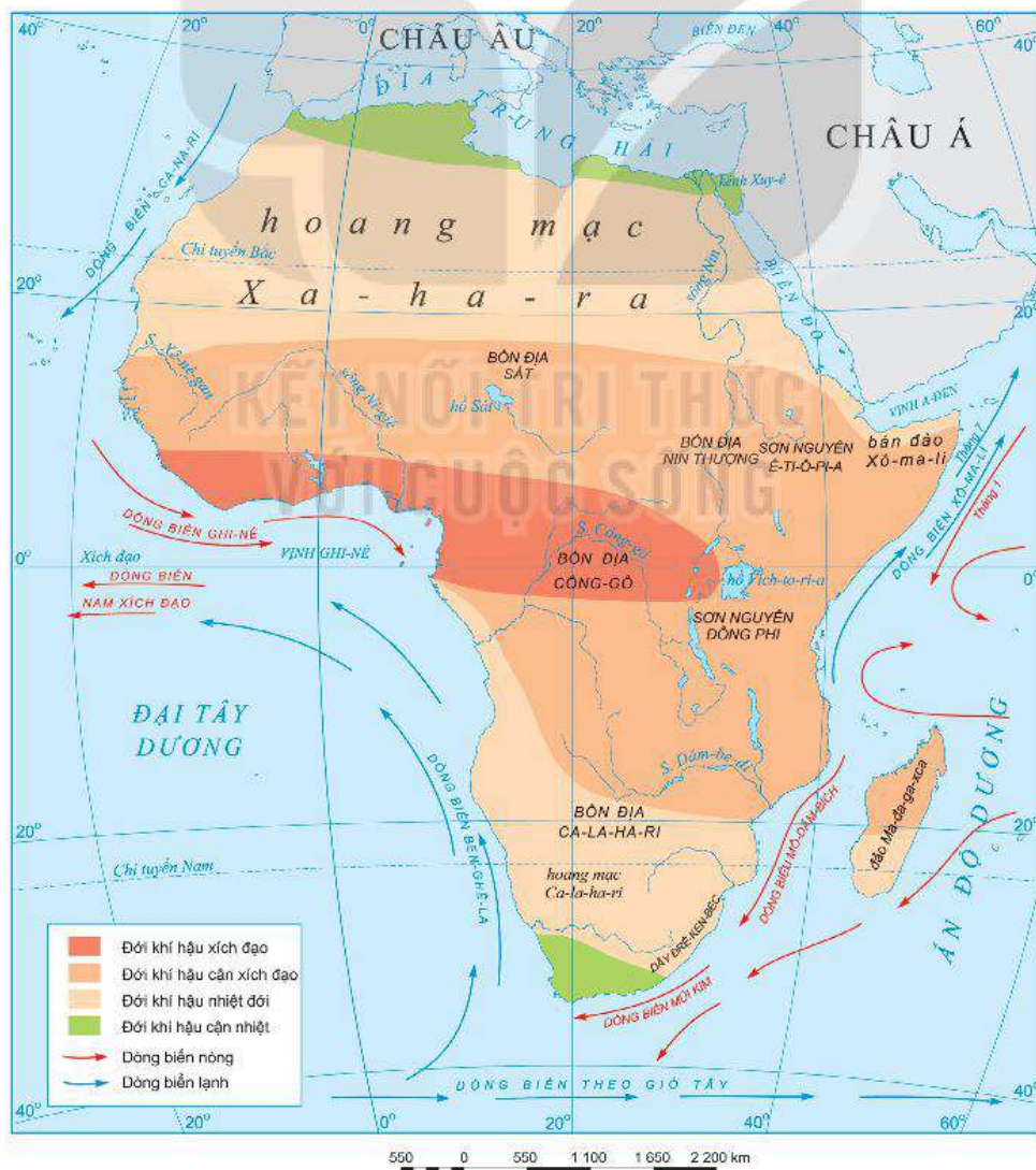
Hình 2. Bản đồ các đới khí hậu ở châu Phi
