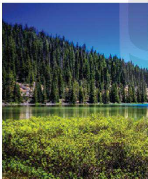
Hình 4. Rừng lá kim ở Hoa Kỳ
