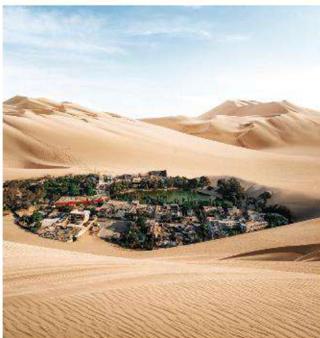
Hình 3. Một ốc đảo ở phía bắc Ma-rốc
