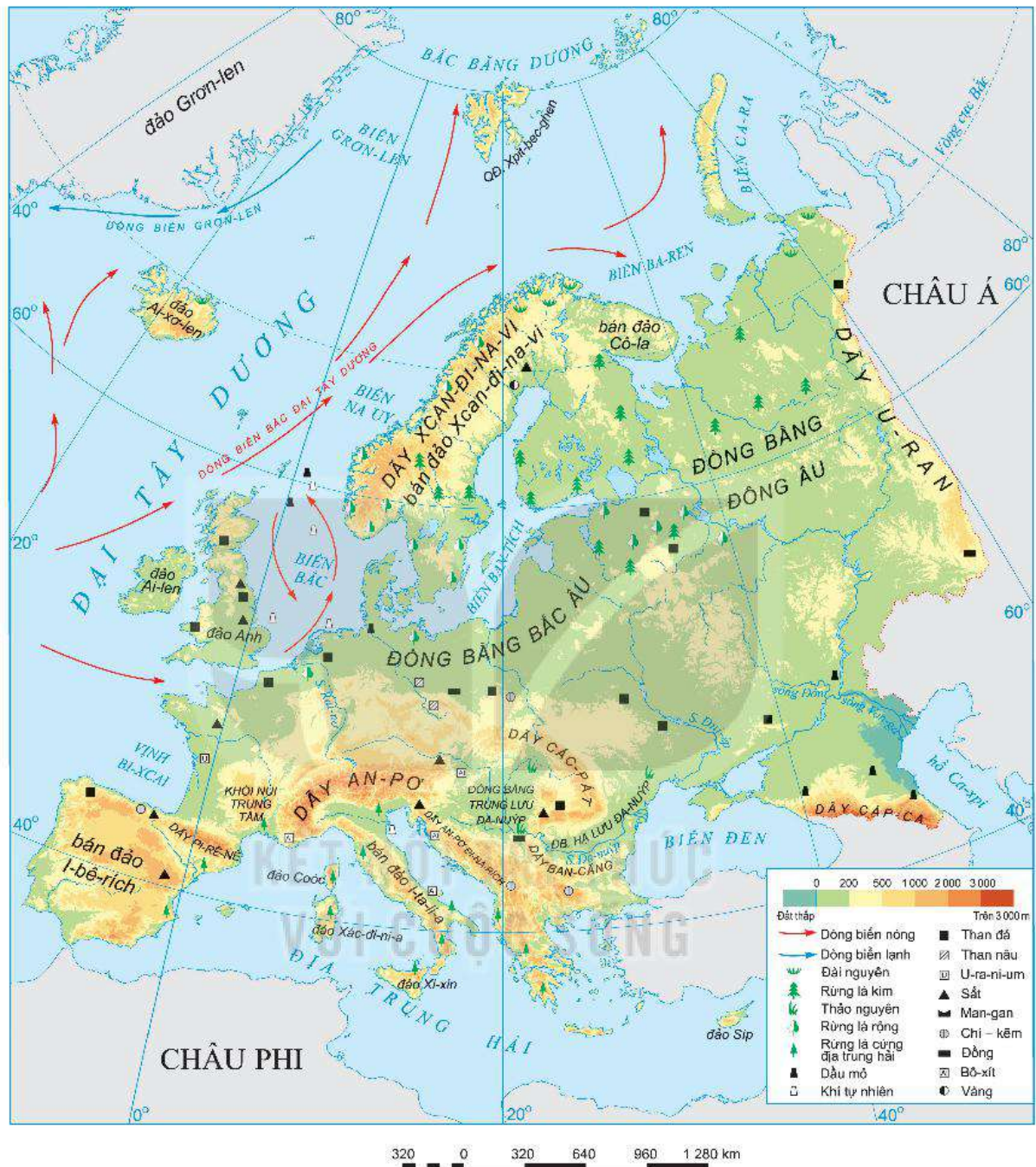
Hình 1. Bản đồ tự nhiên châu Âu
