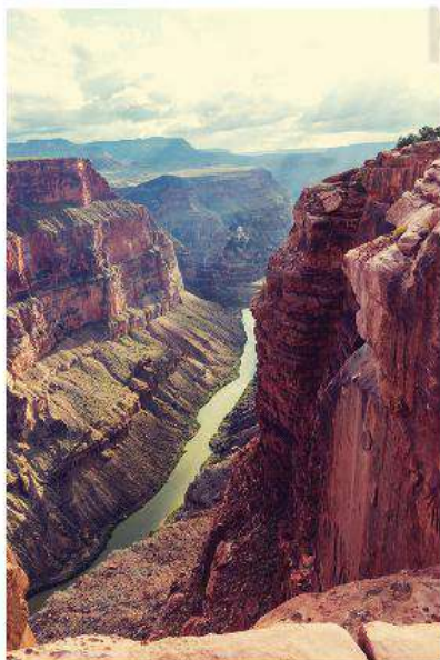
Hình 1. Gran Ca-ny-on, Hoa Kỳ
