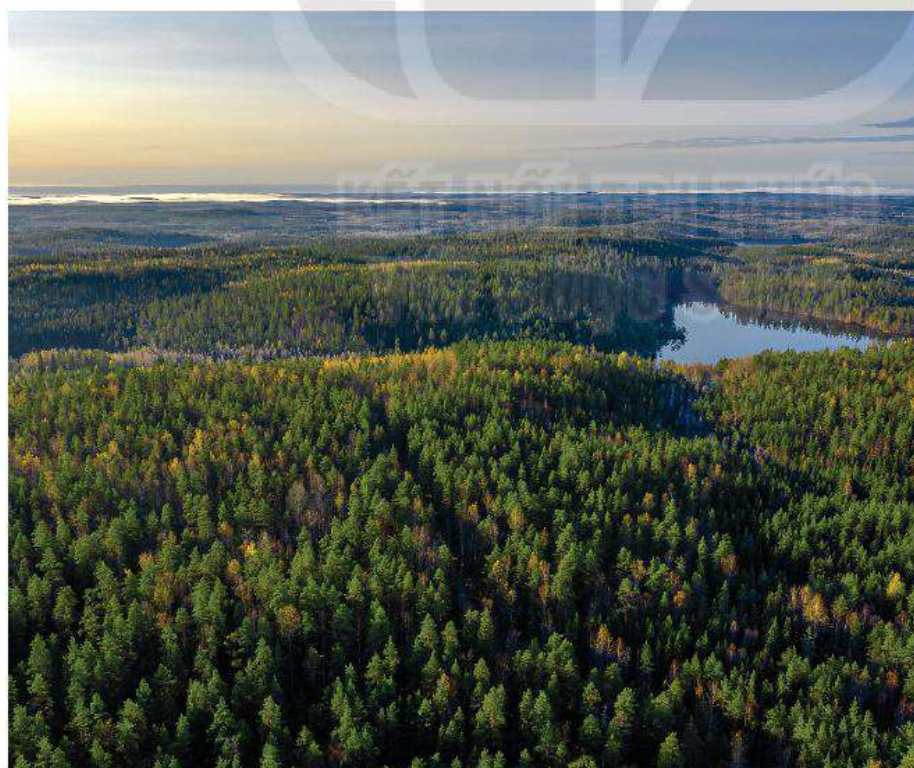
Hình 2. Một khu rừng ở Phần Lan
