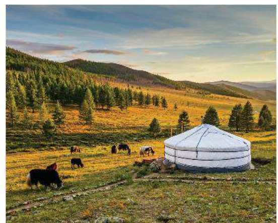
Hình 6. Cảnh quan thảo nguyên rừng ở Mông Cổ
