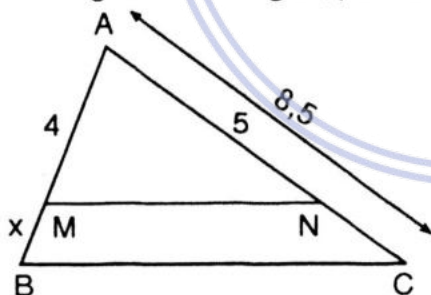
a) MN \parallel BC
