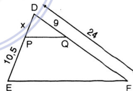
b) PQ \parallel EF
