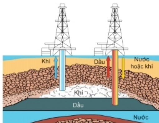
Hình 14.2 Cấu trúc mỏ dầu
