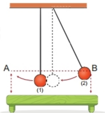
Hình 48.5 Thí nghiệm về sự bảo toàn năng lượng
