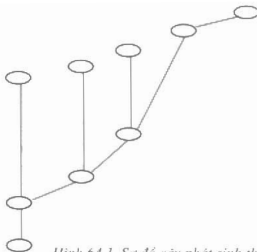
Hình 64.1. Sơ đồ cây phát sinh thực vật
