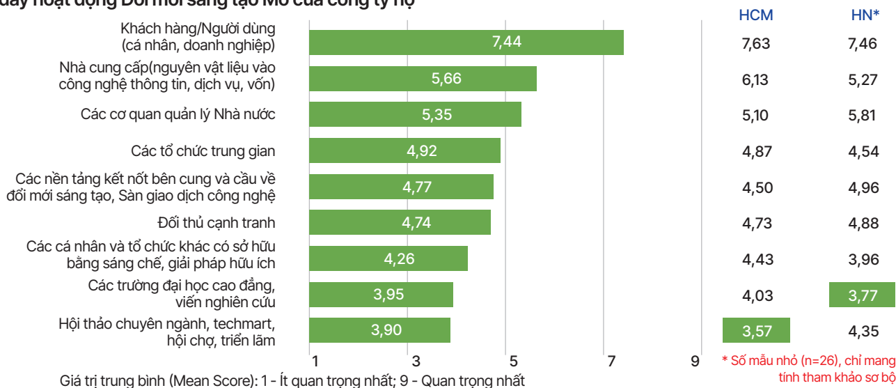
Biểu đồ 6: Mức độ quan trọng của các nguồn hỗ trợ, thúc đẩy Đổi mới sáng tạo Mở
