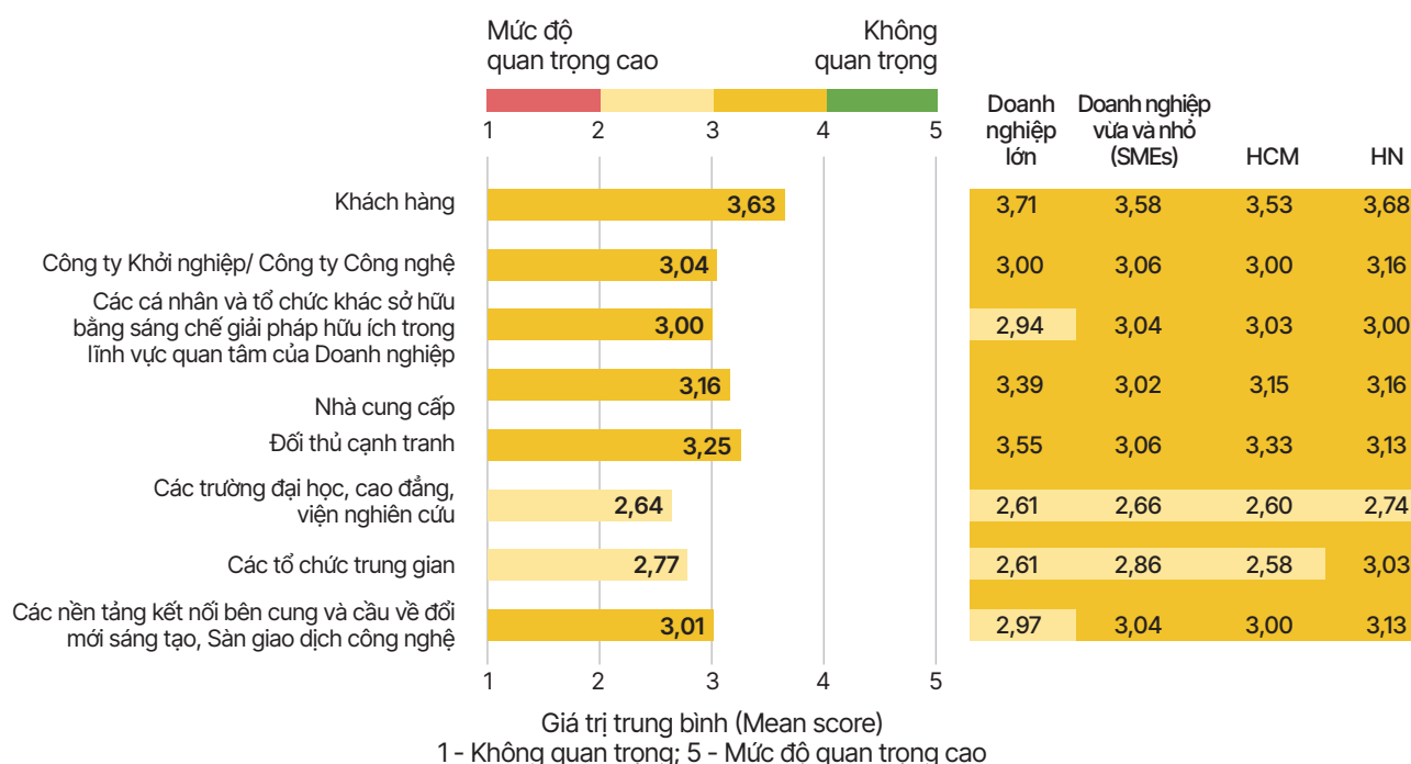
Biểu đồ 11: Mức độ quan trọng của các nhóm đối tác trong các hoạt động Đổi mới sáng tạo Mở của Doanh nghiệp
