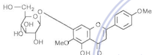
Pectolarigenin - 7 - O - \beta - D - glucosid
