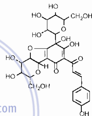
Safflor yellow A
