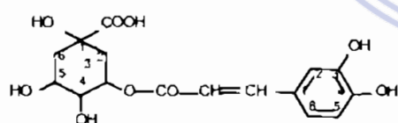
Acid clorogenic (= acid cafeyl - 3 quinic) chính tên
