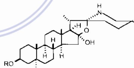
Soladulcin
