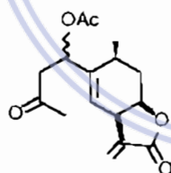
Xanthumin
