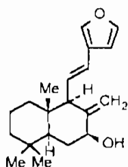
Coronarin A
