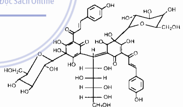
Safflor yellow B
