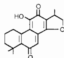
Miltionon II
