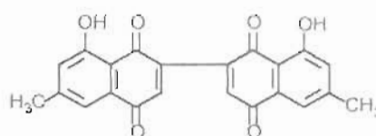
Mamegakinon
