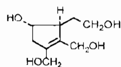
Eucomiol
