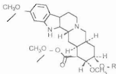
Yohimbin
