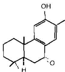
Nimbiol
