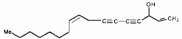
Panaxynol
