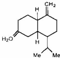
\epsilon -Muurolen
