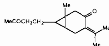
Curcolon (Nhóm eudesman)
