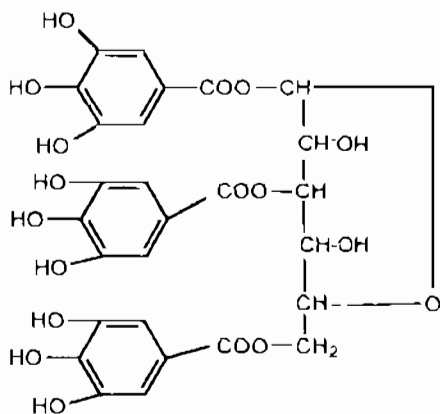
Corilagin
