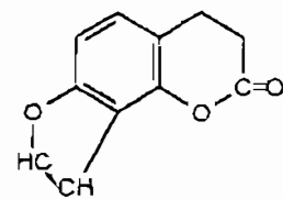
(3) isopsoralen (anglicin)
