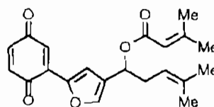
1,1-Benzoquinon analog của shikonofuran
