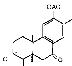
Nimbiin
