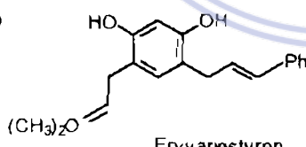
Eryvanestyren
