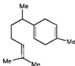
(12) \beta curcumen
