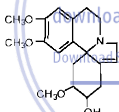
Erytratidin
