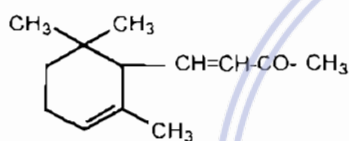
\alpha ionon
