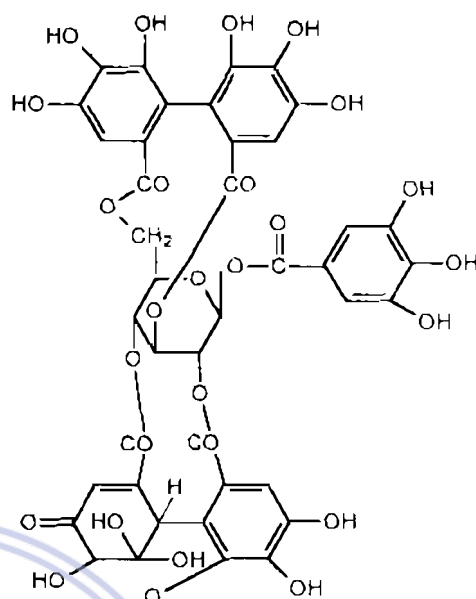
Geraniin
