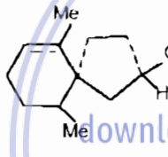
Hinesol
