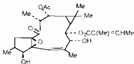
3, 12 - di - O - acetyl - 8 - O - Tigloylingol
