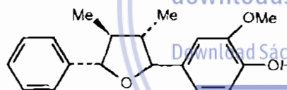
Fragransin A 2
