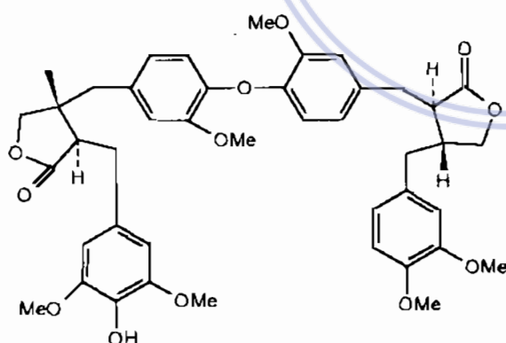
Neosartichin A
