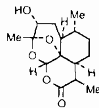
Qinghaosu IV
