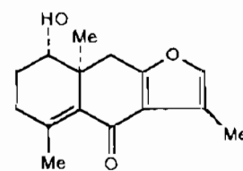
Curcolon (Nhóm eudesman)
