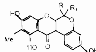
Boeravinon D. RH , R_1 = OMe
