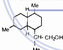
Artemisinol
