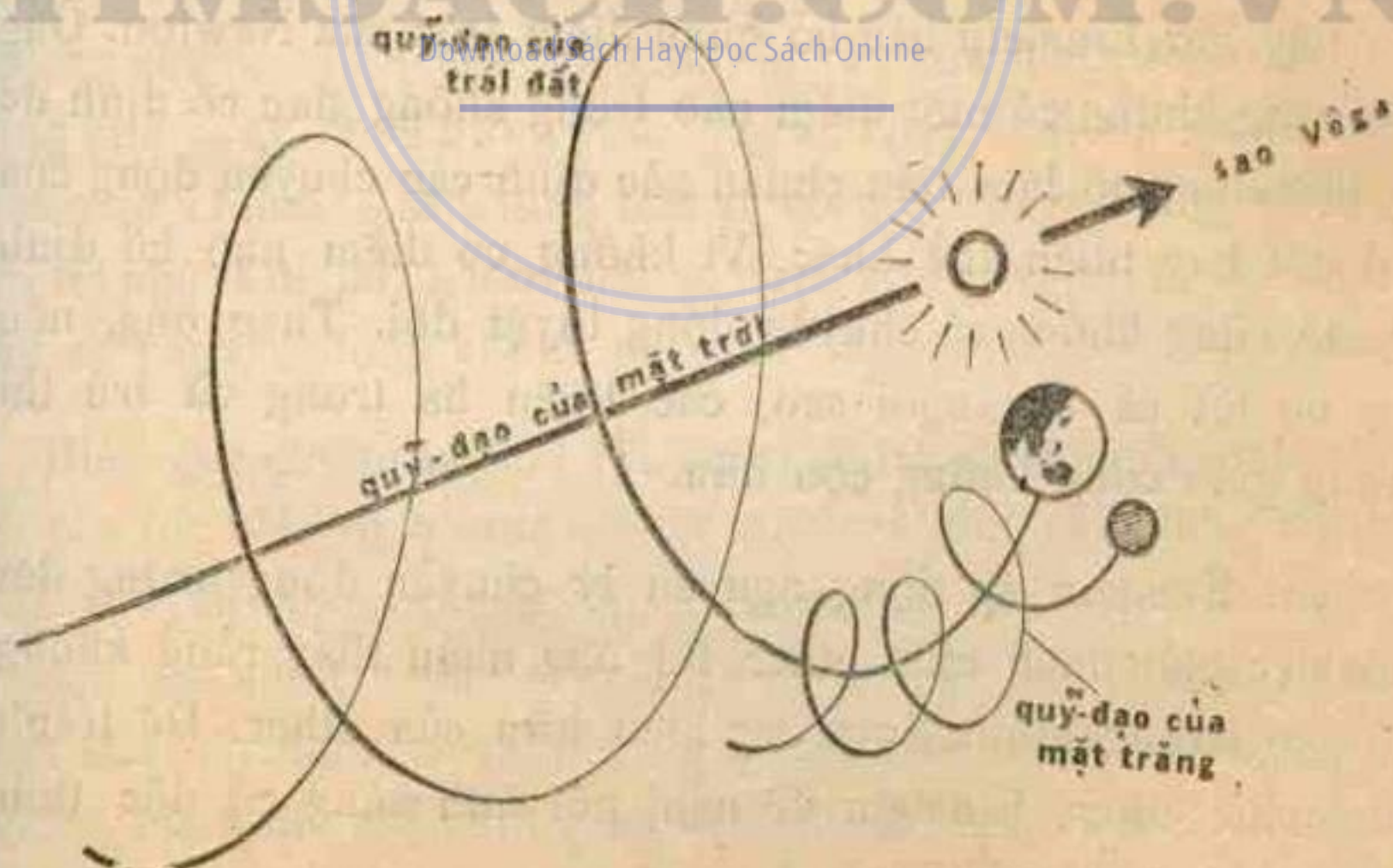
Chuyển động tương đối của mặt trăng, trái đất và mặt trời trong không gian.
