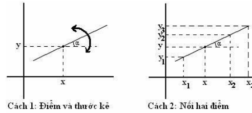
Hình 10: Các cách vẽ đường thẳng trên nguyên tắc
