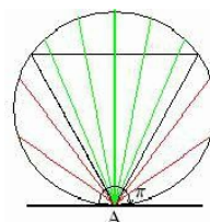
Hình 7: Nghịch lý Bertran 1
