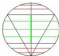
Hình 9: Nghịch lý Bertrand 3
