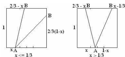
Hình 18: Trường hợp các điểm cắt ngẫu nhiên.
