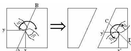
Hình 20: Bê. Bánh tách ra hai phần. Sau đó chọn một phần để bê tiếp. Đếm bê trong bánh và vết cắt ở bất kỳ đâu.
