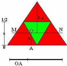
Hình 6: Minh họa bẻ que 2
