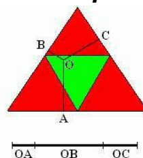
Hình 5: Minh họa bẻ que
