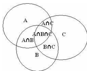
Hình 21: Biểu đồ Venn.
