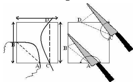
Hình 19: Cắt bằng lạt và bằng dao. Bánh dẻ nguyên khối cắt xong đường cắt sau. Vết cắt thứ hai không được chồng lên vết đầu.
