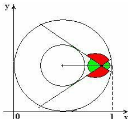
Hình 13: Nghịch lý Bertrand. Điểm bên trong và thước kẻ.
