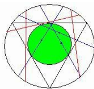
Hình 8: Nghịch lý Bertrand 2
