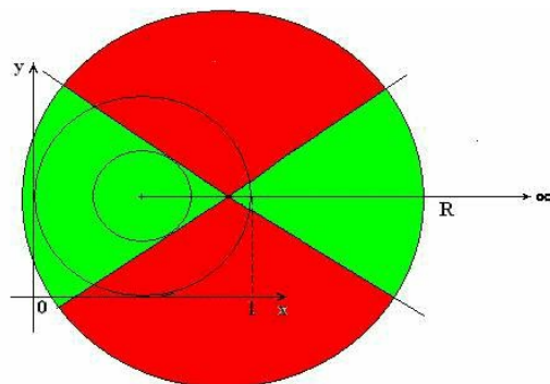
Hình 14: Điểm bên trong điểm bên ngoài. Dù R tiến đến đâu, tỷ lệ giữa màu xanh với phần tổng đều bằng góc giữa hai tiếp tuyến của \pi .
