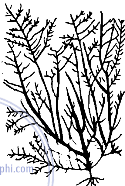
Hình 358. Thạch hoa thái - Gelidium amansii
