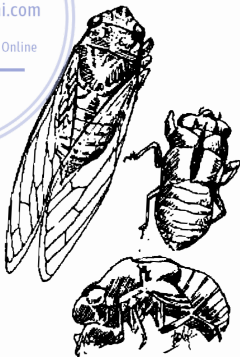
Hình 617. Thuyền thuế - Cryptotympana pustulata và Periostracum cicadae
