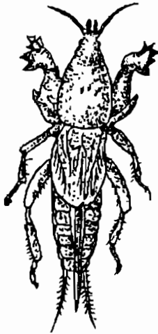
Hình 727. Con dế - Gryllotalpa unispinalpa
