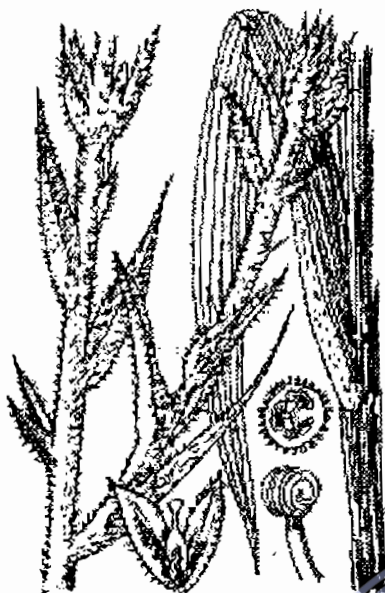
Hình 22. Cỏ đuôi lương Philydrium lanuginosum
