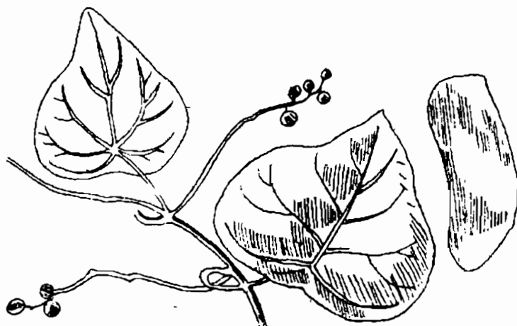
Hình 394. Phần phòng kỷ - Stephania tetrandra
