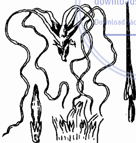
Hình 458. Sừng dê hoa đỏ - Strophanthus robustus
