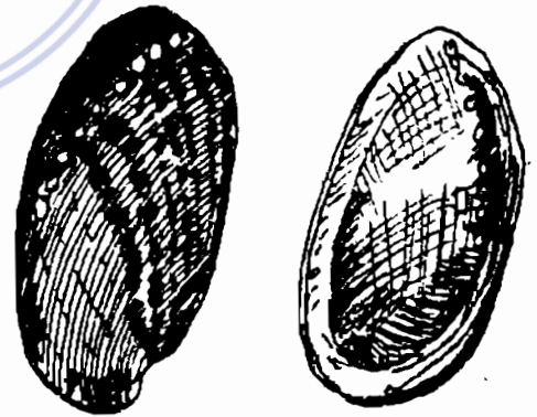
Hình 373. Thạch quyết minh - Concha Halitidis
