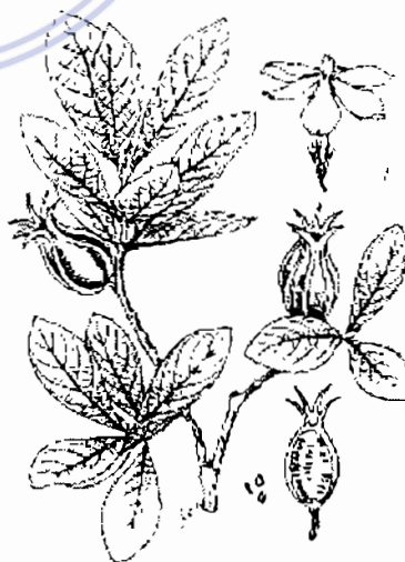
Hình 167. Dành dành - Gardenia jasminoides 1. Cành có hoa, quả; 2. Quả bổ dọc
