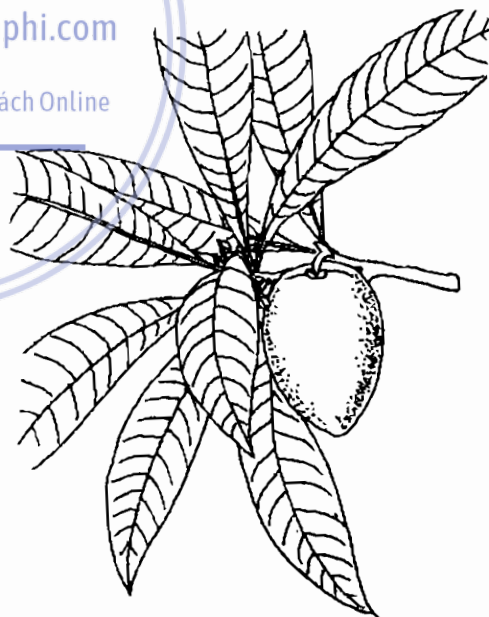
Hình 701. Lêkima - Lucuma mammosa
