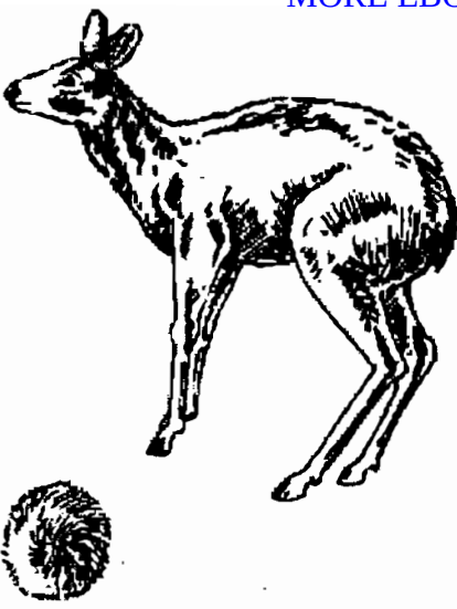
Hình 739. Hươu xạ và túi xạ - Moschus moschiferus
