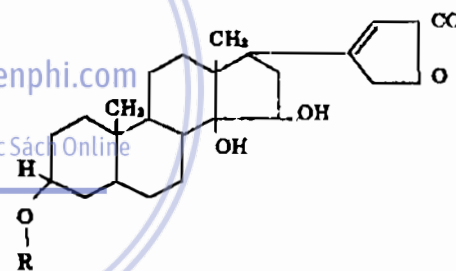
Rodexin B=R là l. ramnoza
