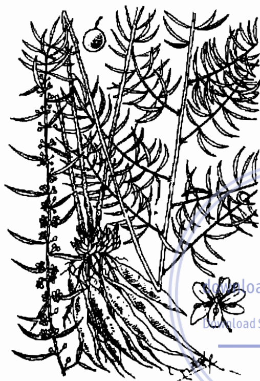
Hình 551. Thiên môn đông- Asparagus cochinchinensis
