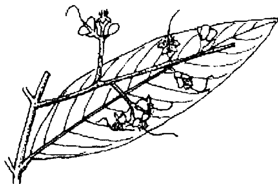
Hình 155. Săng lễ - Lagerstroemia calyculata
