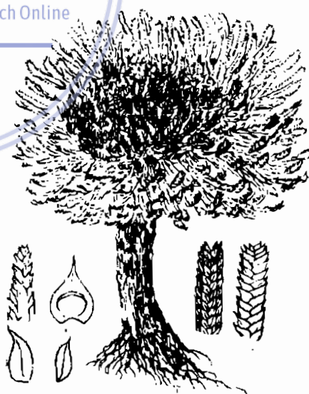
Hình 207. Móng lương rồng - Selaginella tamariscina
