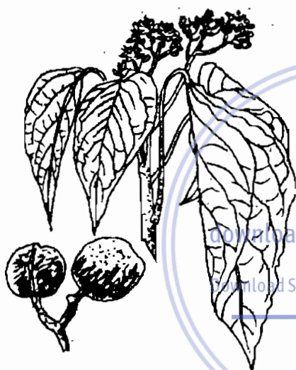
Hình 363. Cây lai - Aleurites moluccana
