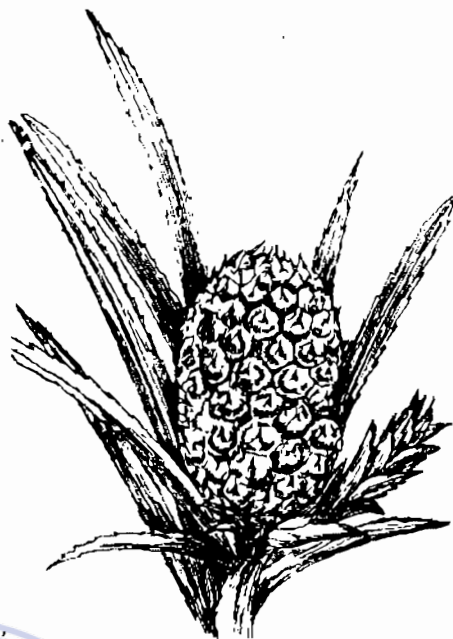
Hình 197. Dứa - Ananas sativa
