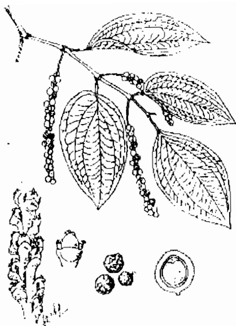
Hình 278. Hồ tiêu - Piper nigrum
