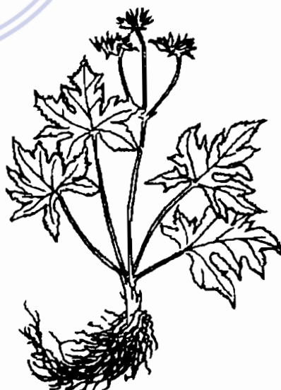
Hình 131. Hoàng liên - Coptis teeta
