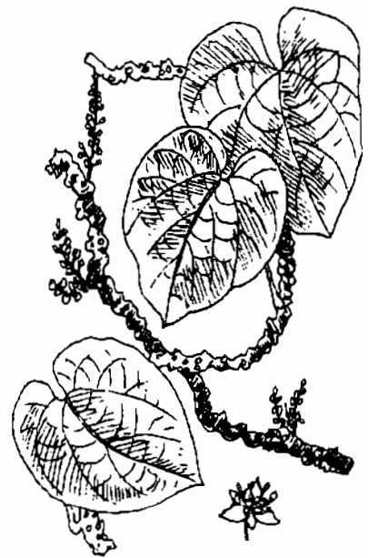
Hình 480. Dây ký ninh - Tinospora crispa
