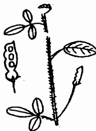
Hình 109. Hàn the - Desmodium heterophyllum
