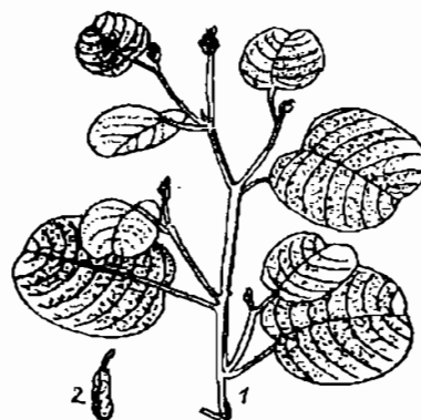
Hình 205. Kim tiền thảo - Desmodium styracifolium 1. Cành 2. Quả
