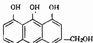
Bachaloin (dự kiến)
