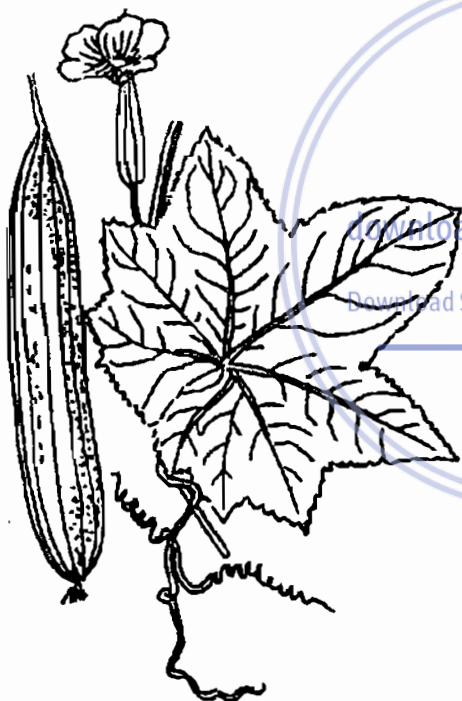
Hình 25. Mướp - Luffa cylindrica
