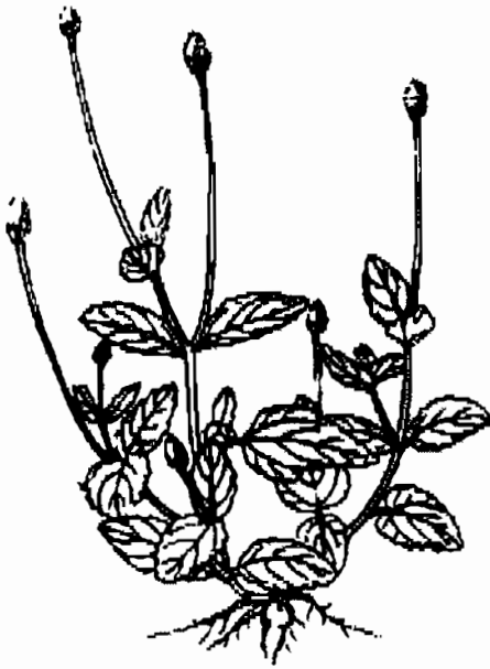
Hình 443. Cúc áo - Spilanthes acmella
