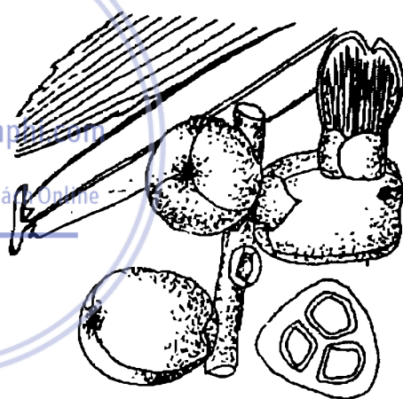
Hình 524. Bụng báng - Arenga saccharifera
