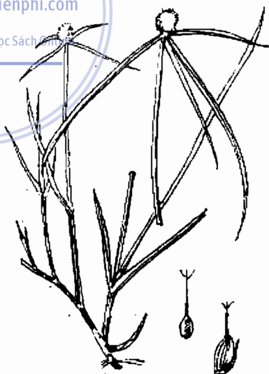
Hình 434. Cỏ bạc đầu - Kyllinga monocephala
