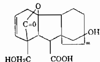
Canavalia giberellin II
