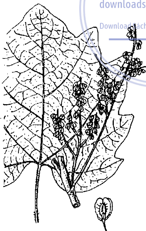
Hình 349. Được dụng đại hoàng - Rheum officinale
