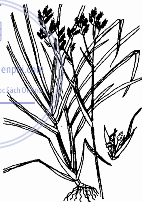
Hình 530. Sả - Cymbopogon nardus
