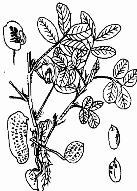
Hình 366. Lạc - Arachis hypogaea
