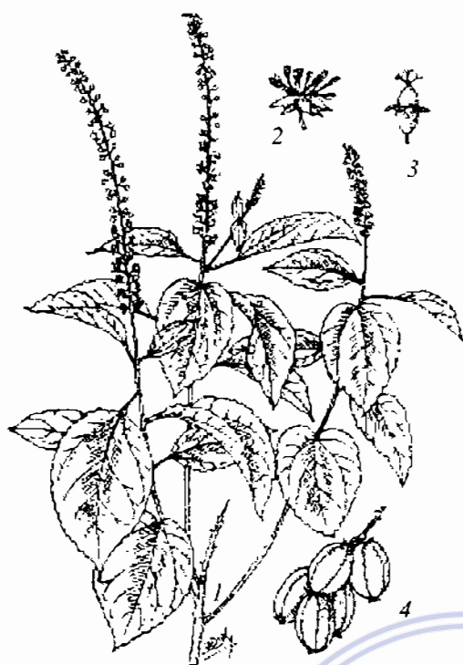
Hình 346. Ba đậu - Croton tiglium
