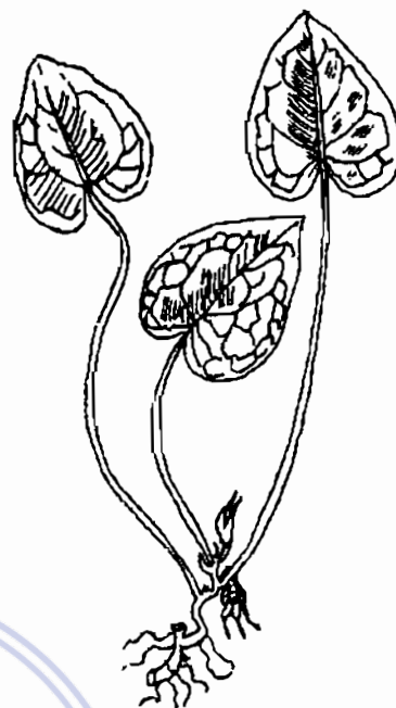
Hình 578. Biến hoá - Asarum caudigerum
