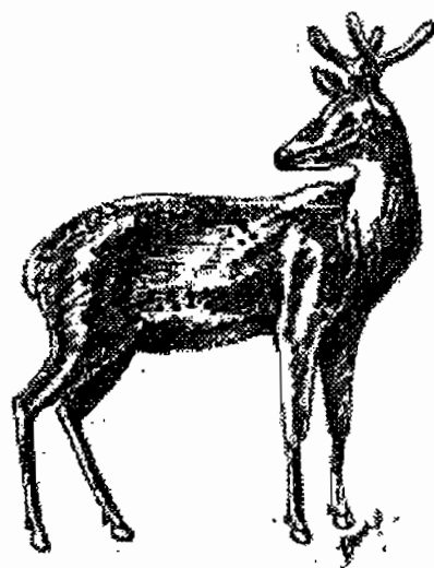
Hình 711. Con hươu sao - Cervus nippon
