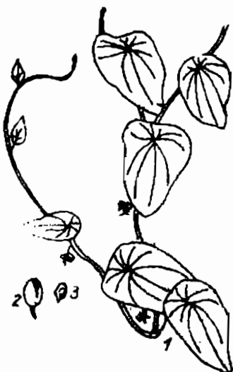
Hình 179. Lỗi tiền - Stephania longicaulis 1. Cành; 2. Quả; 3. Hạt
