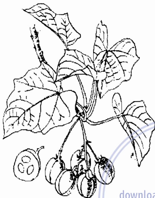
Hình 362. Đậu cọc rào - Jatropha curcas .
