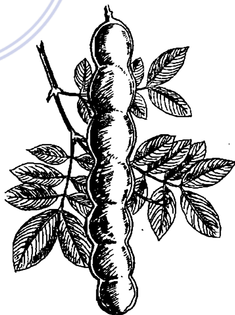
Hình 523. Bàm bàm - Entada phaseoloides
