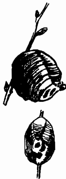
Hình 558. Tang phiêu tiêu - Ootheca Mantidis
