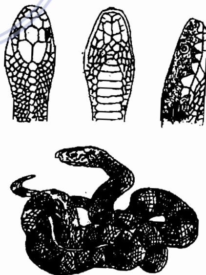
Hình 738. Cạp nong - Bungarus fasciatus
