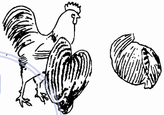
Hình 272. Kê nội kim - Corium Stomachichum
