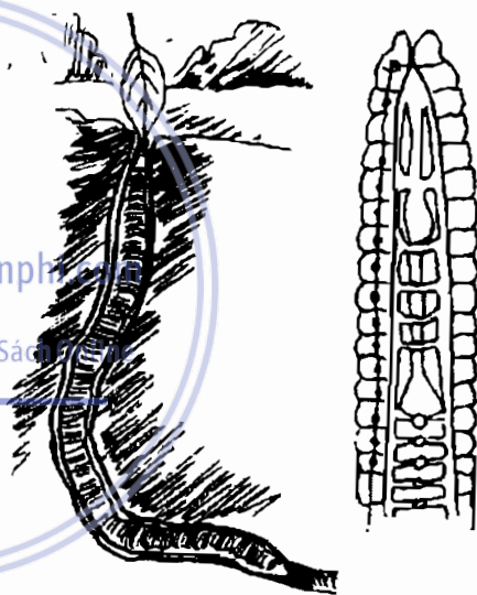
Hình 728. Giun đất - Pheretima asiatica
