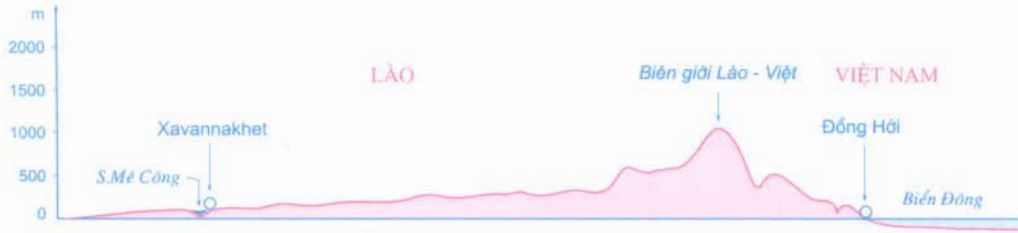
ĐỊA HÌNH TRƯỜNG SƠN BẮC: LÁT CẮT QUA XAVANNAKHET ĐẾN ĐỒNG HỚI
