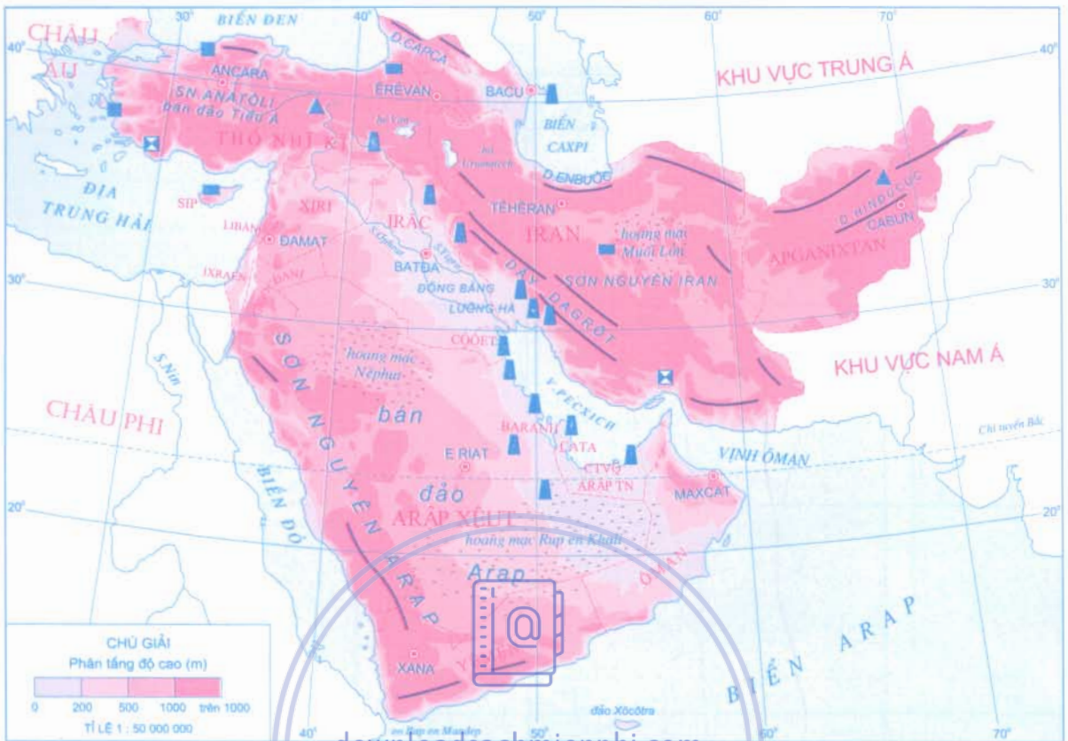
downloadsachmienphi.com Lược đồ Địa hình và khoáng sản khu vực Tây Nam Á
