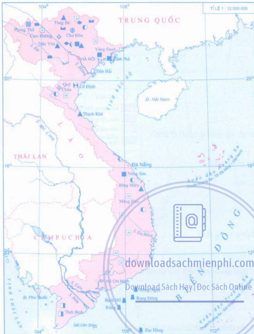
Lược đồ Khoáng sản Việt Nam
