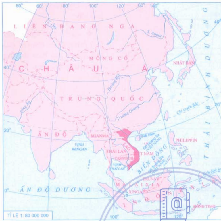
Lược đồ Vị trí Việt Nam trong châu Á
