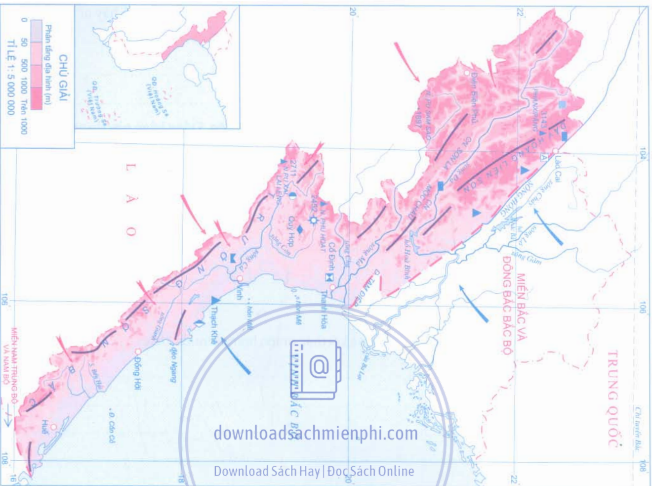
Lược đồ Địa hình và khoảng sân miền Tây Bắc và Bắc Trung Bộ
