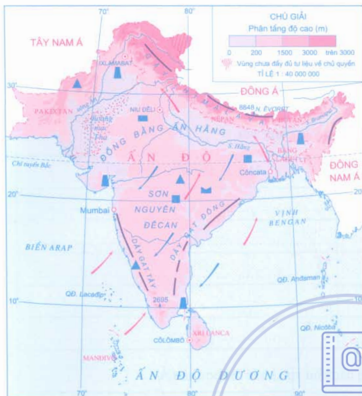
Lược đồ Tự nhiên khu vực Nam Á
