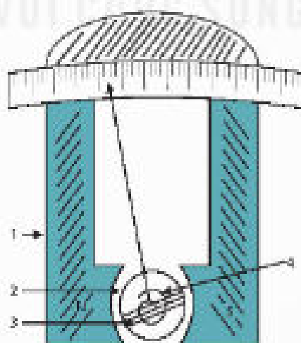
Hình 1.1. Sơ đồ cấu tạo điện kế khung quay
