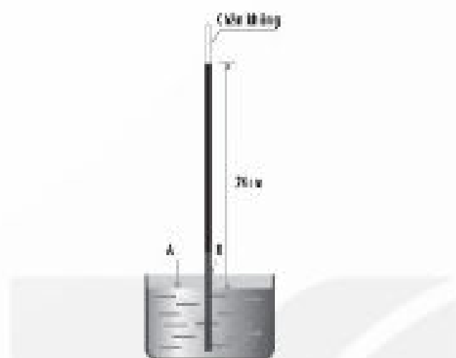
Hình 16.1. Thí nghiệm của Torricelli
