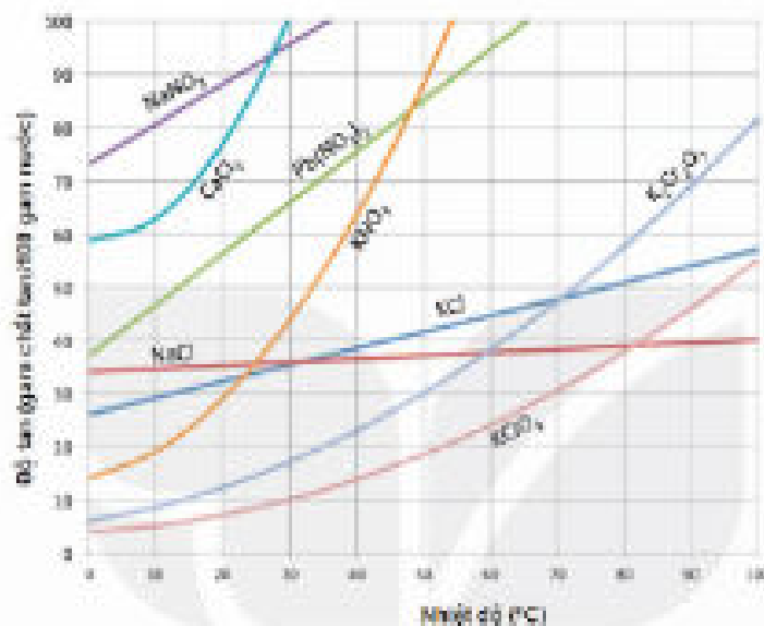
Hình 4.1. Ảnh hưởng của nhiệt độ tới độ tan của một số chất rắn
