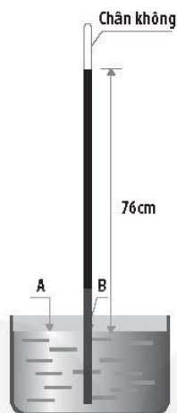
Hình 16.1. Thí nghiệm của Torricelli
