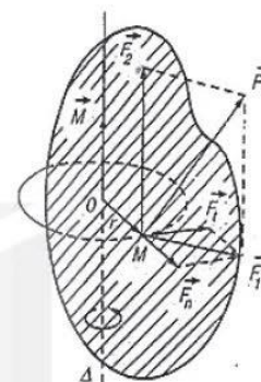
Hình 18.2. Tác dụng của lực trong chuyển động quay
