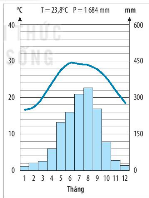
Hình 3. Biểu đồ nhiệt độ và lượng mưa của trạm khí tượng Láng (Hà Nội, Việt Nam)
