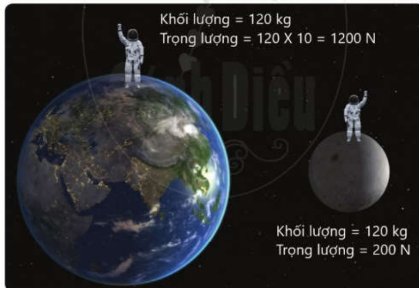
Hình 29.1. Sự khác nhau về cường độ trường hấp dẫn ở mặt đất và ở Mặt Trăng
