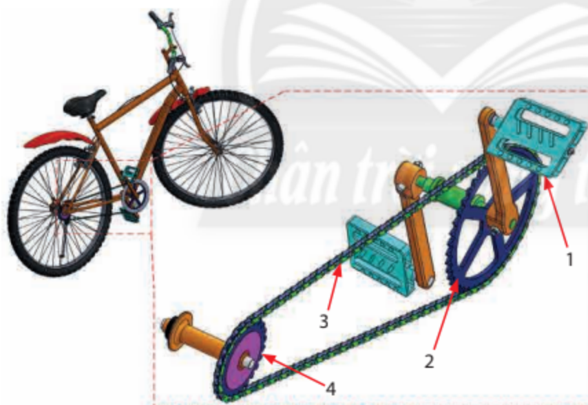
Hình 6.2. Truyền chuyển động trên xe đạp (1) Bàn đạp; (2) Đĩa xích; (3) Dây xích; (4) Líp
