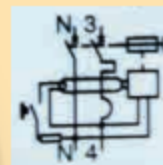
Hình 8.4. Kí hiệu Aptomat chống giật
