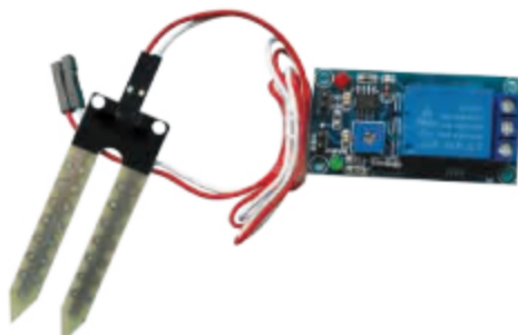
b) Mô đun cảm biến độ ẩm
