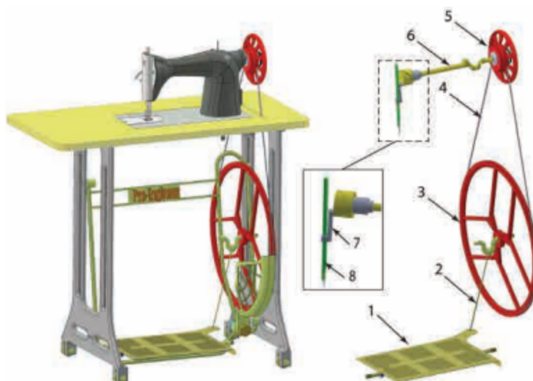
Hình 6.8. Máy may đạp chân:
