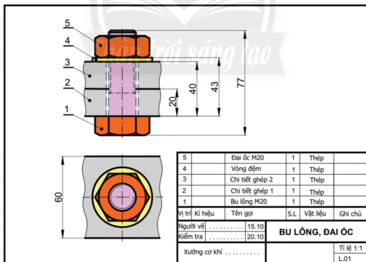
Hình 3.3. Bản vẽ lắp bu lông, đai ốc
