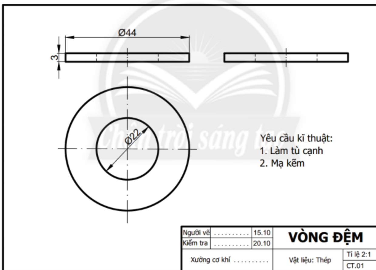
Hình 3.2. Bản vẽ chi tiết vòng đệm
