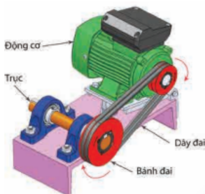
Hình 6.1. Động cơ điện
