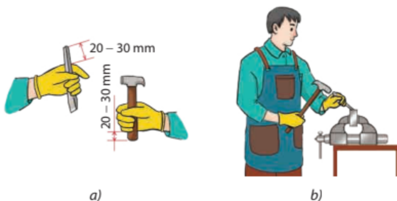
Hình 5.7. Cách cầm đục, búa và tư thế đục
