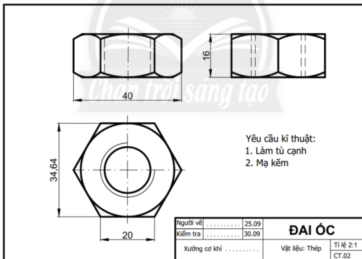
Hình 3.5. Bản vẽ chi tiết đai ốc
