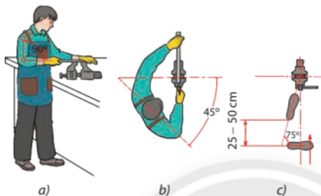
Hình 5.9. Cách cầm dũa và thao tác dũa
