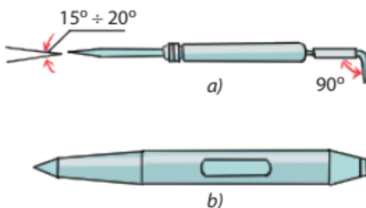
Hình 5.7. Dụng cụ vạch dấu
