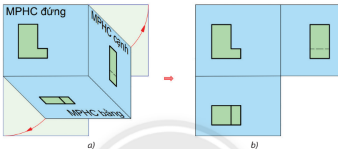
Hình 2.5. Mở các mặt phẳng hình chiếu
