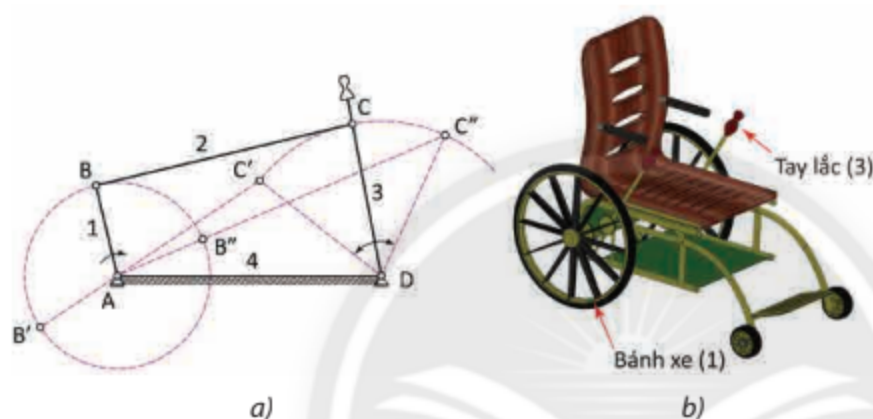
Hình 6.7. Cơ cấu tay quay thanh lắc (a)
