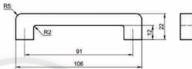
Hình 1.6. Ứng dụng một số loại nét vẽ
