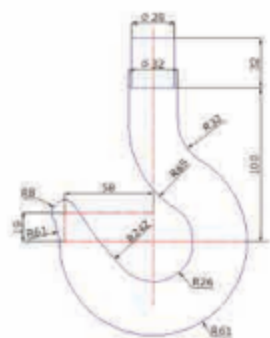
a) Hình vẽ thiết kế
