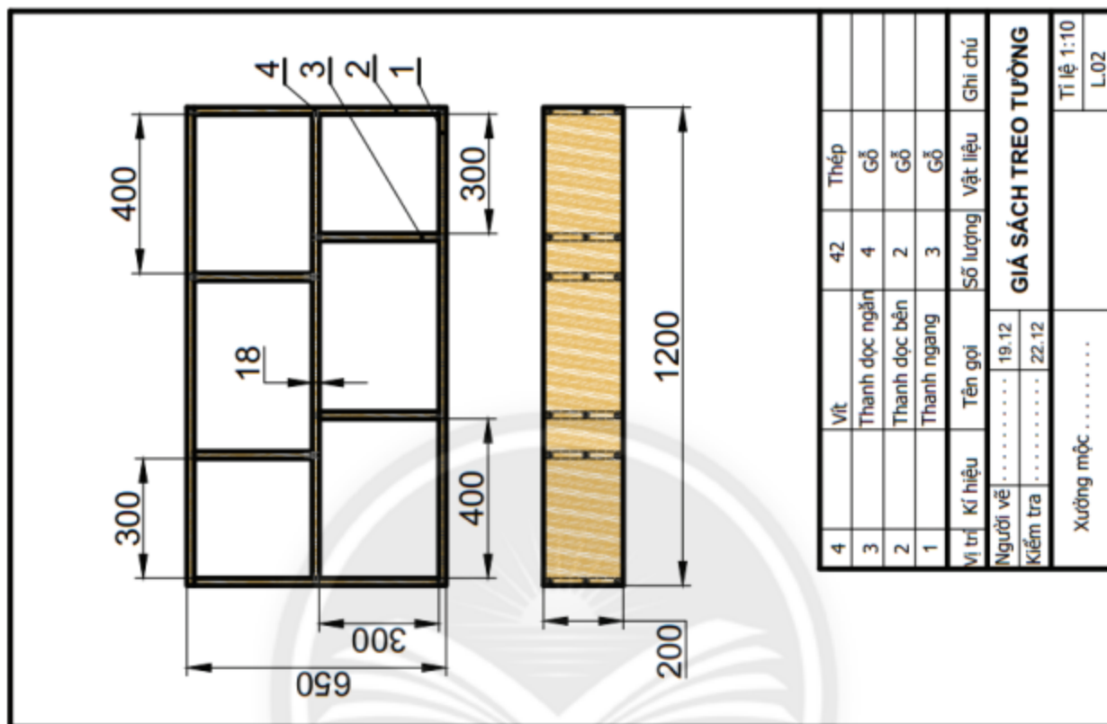
Hình 3.7. Bản vẽ giá sách treo tường
