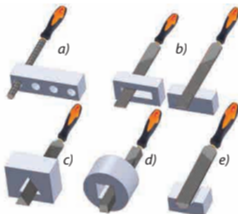
Hình 5.8. Các loại dũa
