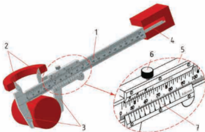
Hình 5.3. Thước cặp
