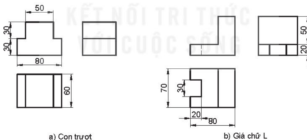
Hình 2.5. Các hình chiếu vuông góc của vật thể
