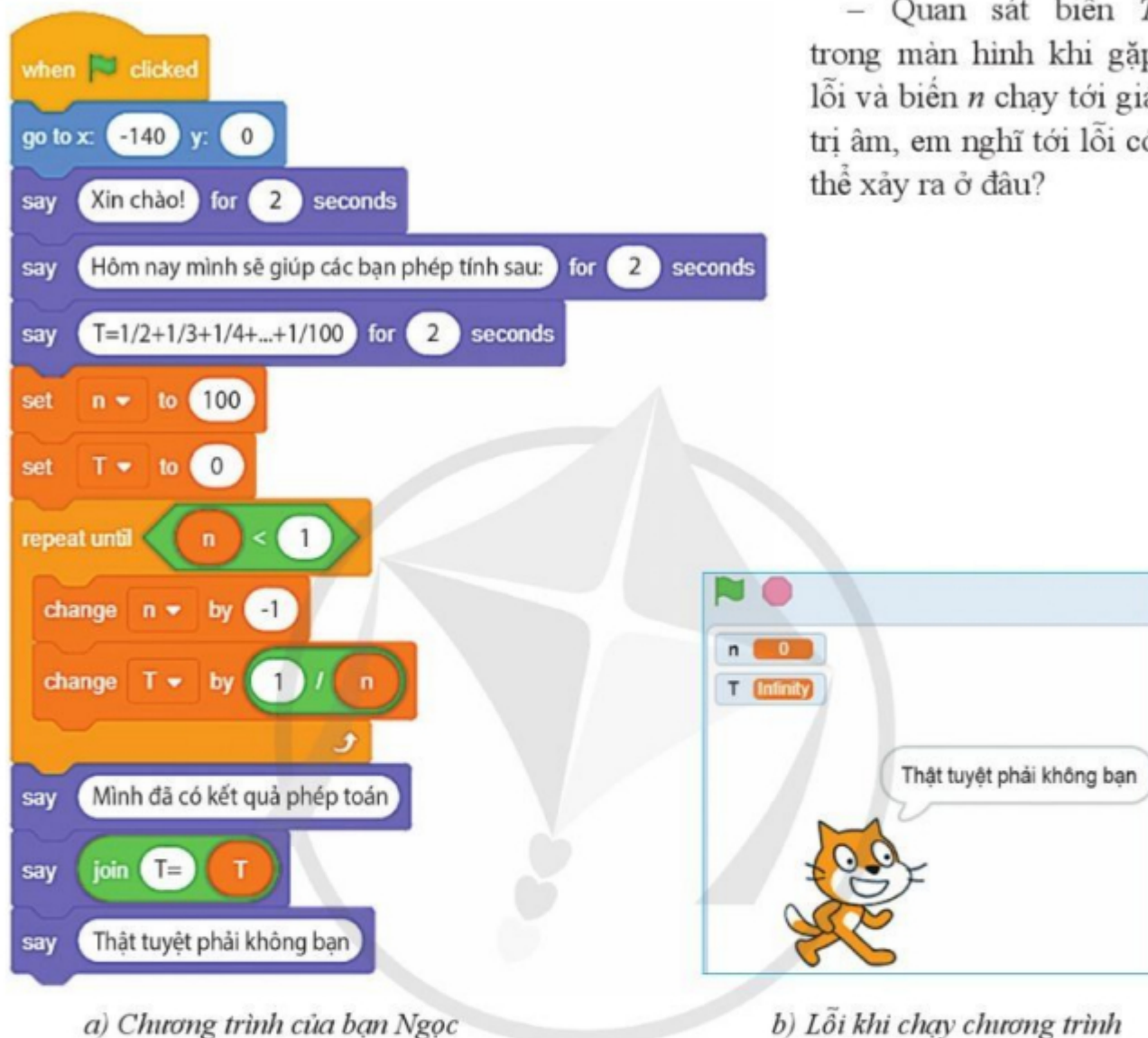
Hình 1. Chương trình còn có lỗi của bạn Ngọc
