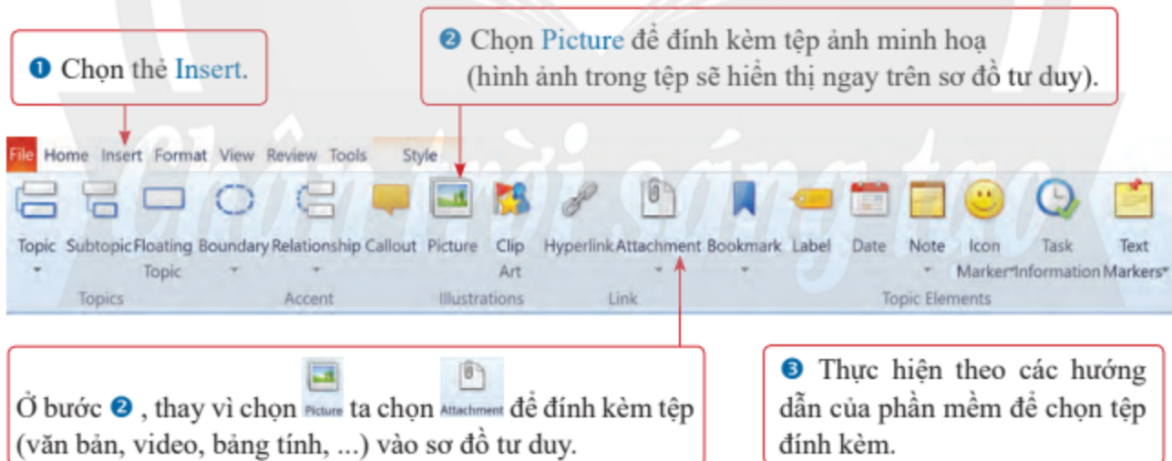
Hình 2. Các bước đính kèm tệp vào sơ đồ tư duy
