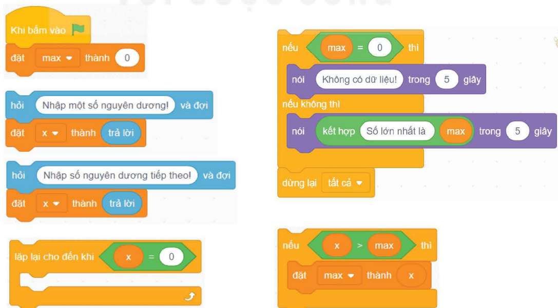
Hình 16.3. Các khối lệnh thành phần của chương trình tìm giá trị lớn nhất
