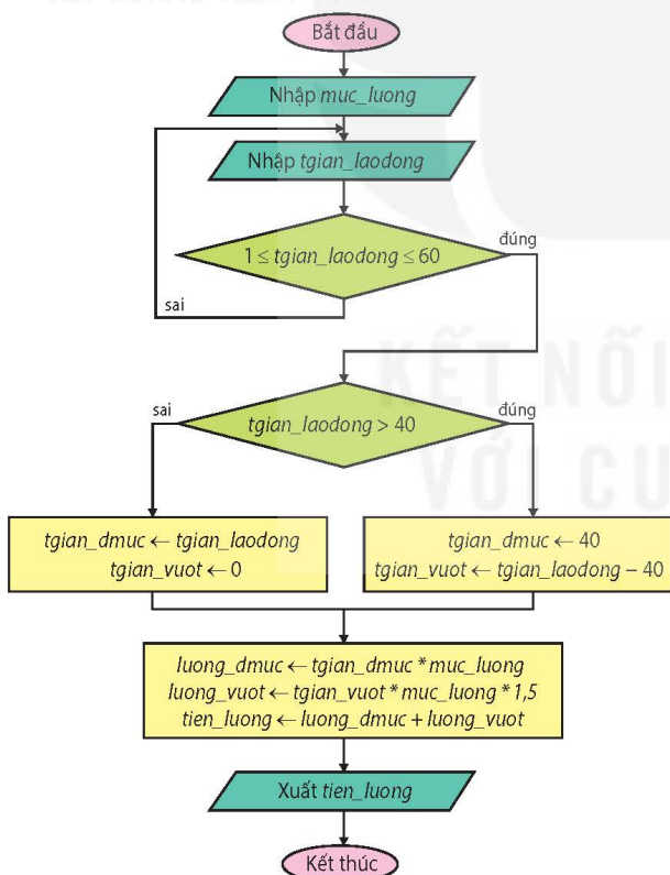
Hình 15.3. Thuật toán tính lương
