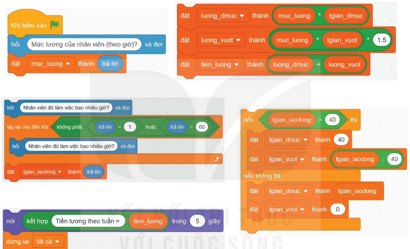
Hình 16.2. Các khối lệnh thành phần của chương trình tính lương
