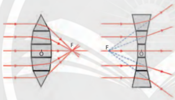
▲ Hình 7.10. Minh họa đường đi của chùm tia sáng song song qua “các lăng kính nhỏ” tạo nên: a) chùm tia hội tụ; b) chùm tia phân kì
