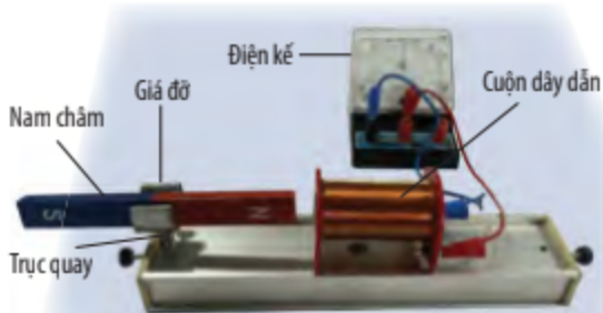
▲ Hình 12.1. Bố trí thí nghiệm dùng nam châm vĩnh cửu để tạo ra dòng điện
