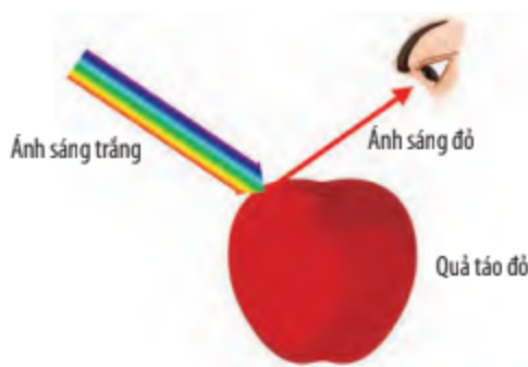
▲ Hình 5.6. Quả táo có màu đỏ dưới ánh sáng trắng
