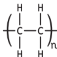
▲ Hình 30.1. Công thức cấu tạo polyethylene
