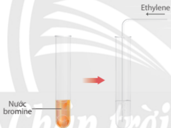
▲ Hình 22.2. Ethylene tác dụng với nước bromine
