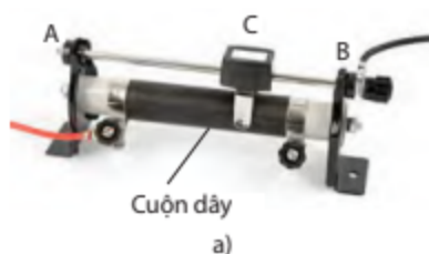
▲ a) Biến trở con chạy; b) Kí hiệu của biến trở trong mạch điện
