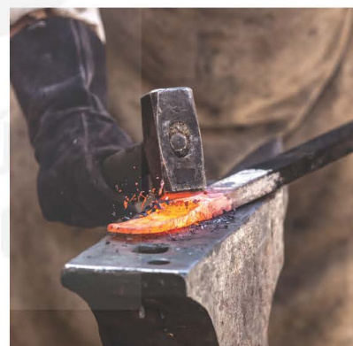
Hình 2.1 Búa chuyển động đập vào thanh thép, làm biến dạng thanh thép
