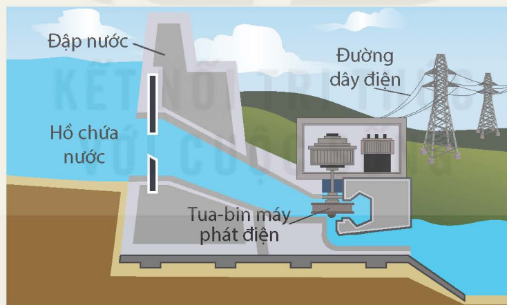
Hình 2.3 Sơ đồ đập thủy điện
