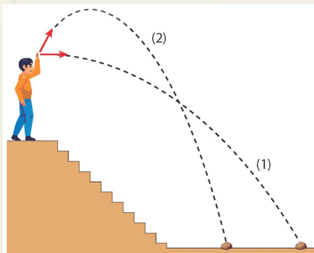
Hình 3.3 Vật được ném từ cùng độ cao với cùng tốc độ ban đầu theo các hướng khác nhau
