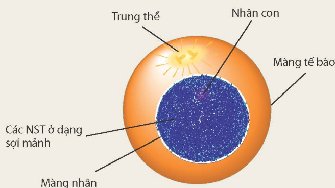
Hình 42.1 Nhiễm sắc thể trong tế bào
