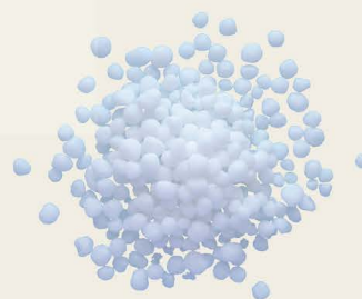
Urea, CO(NH_2)_2 (một loại phân đạm)
