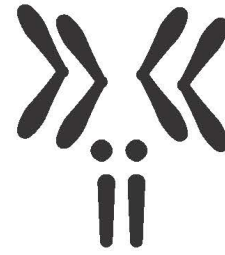
Hình 42.5 Bộ nhiễm sắc thể lưỡng bội ở ruồi giấm cái ( Drosophila melanogaster )
