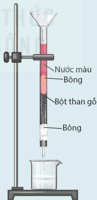
Hình 21.1 Thí nghiệm tìm hiểu tính chất hấp phụ của bột than gỗ
