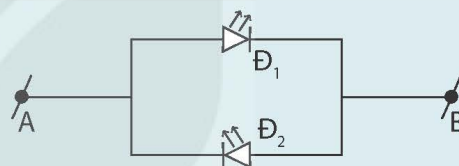
Hình 14.5 Sơ đồ mạch điện gồm hai đèn LED mắc song song, ngược cực
