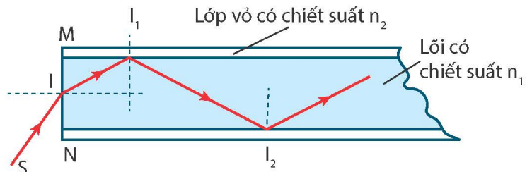
Hình 6.4 Đường truyền của chùm tia sáng trong sợi quang
