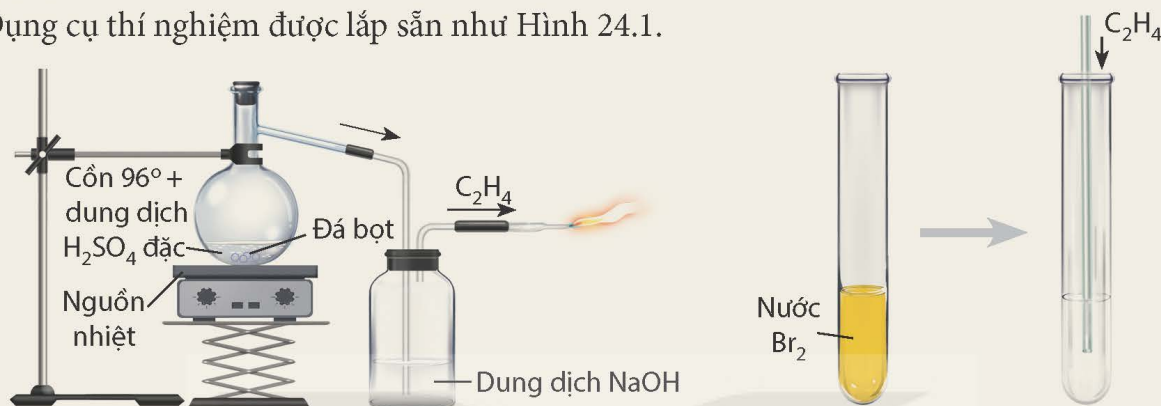
a) Điều chế và đốt cháy ethylene
