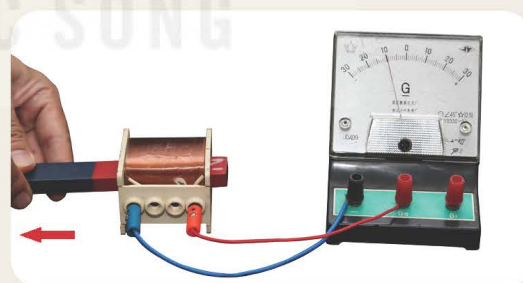
b) Đưa cực Bắc của thanh nam châm vĩnh cửu ra xa cuộn dây dẫn
