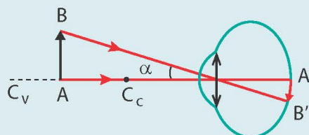
Hình 10.2 Góc trông vật \alpha tạo bởi hai tia sáng xuất phát từ hai điểm A và B tới mắt
