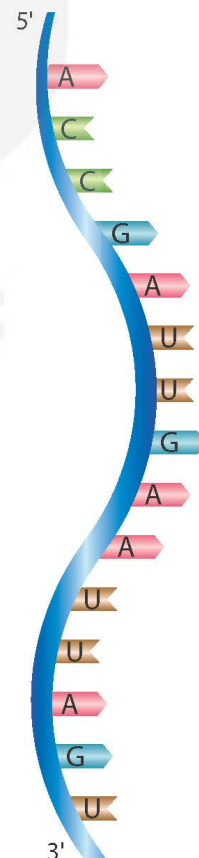
Hình 38.2 Mô hình cấu trúc của đoạn RNA
