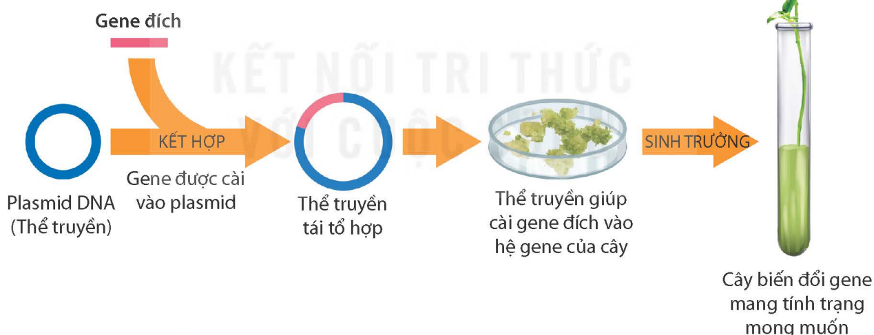
Hình 48.1 Công nghệ tạo giống cây trồng biến đổi gene
