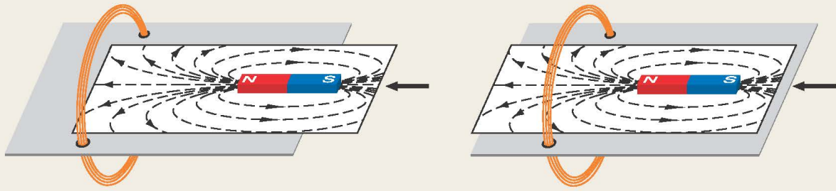
a) Khi nam châm ở xa cuộn dây dẫn
