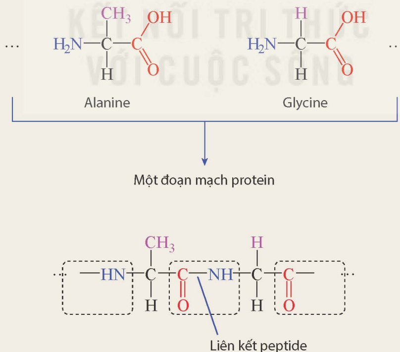
Hình 31.1 Amino acid và protein
