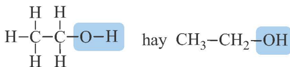
Hình 26.2 Công thức cấu tạo của ethylic alcohol
