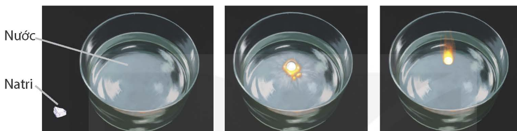
Hình 18.5 Kim loại natri phản ứng với nước
