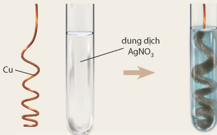
Hình 19.2 Phản ứng của kim loại Cu với dung dịch \text{AgNO}_3
