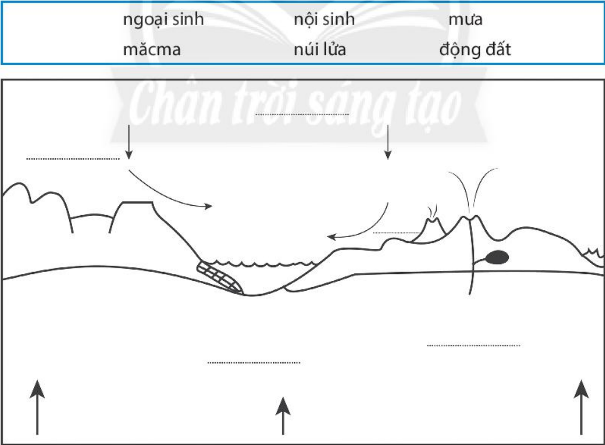
Hình 10.1. Quá trình nội sinh và ngoại sinh
