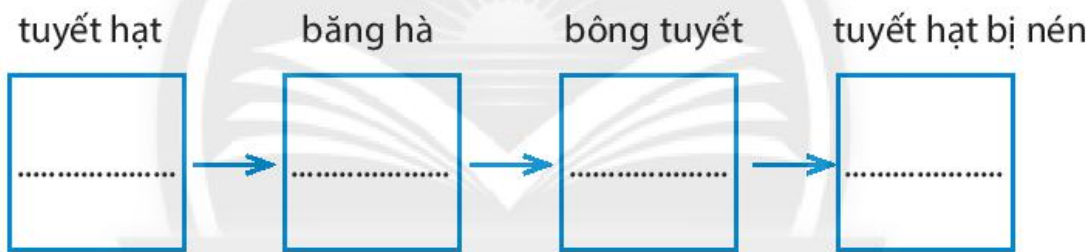
Hình 16.2. Quá trình hình thành băng hà
