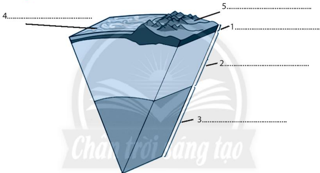
Hình 9.1. Cấu tạo của Trái Đất
