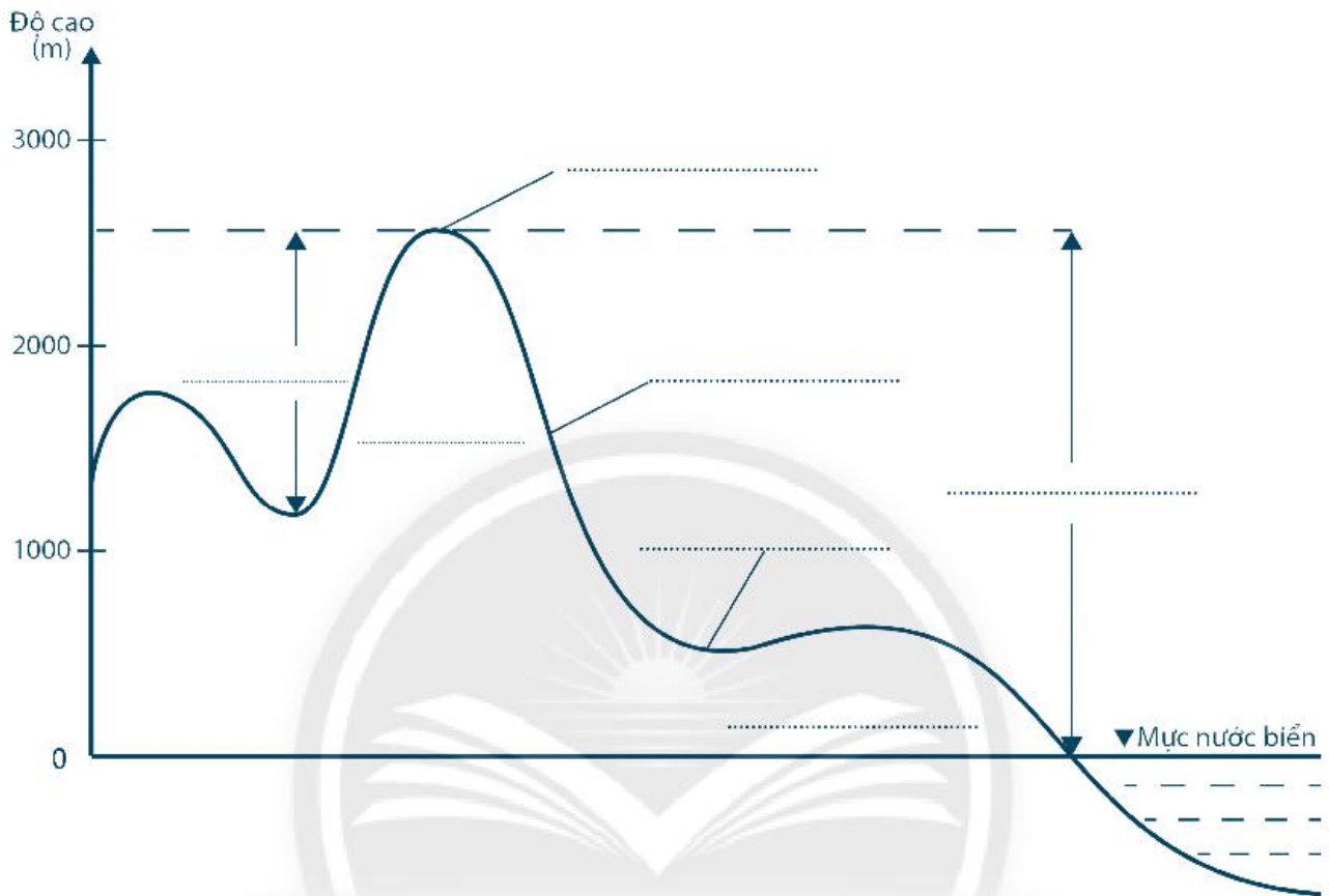
Hình 10.3. Độ cao địa hình
