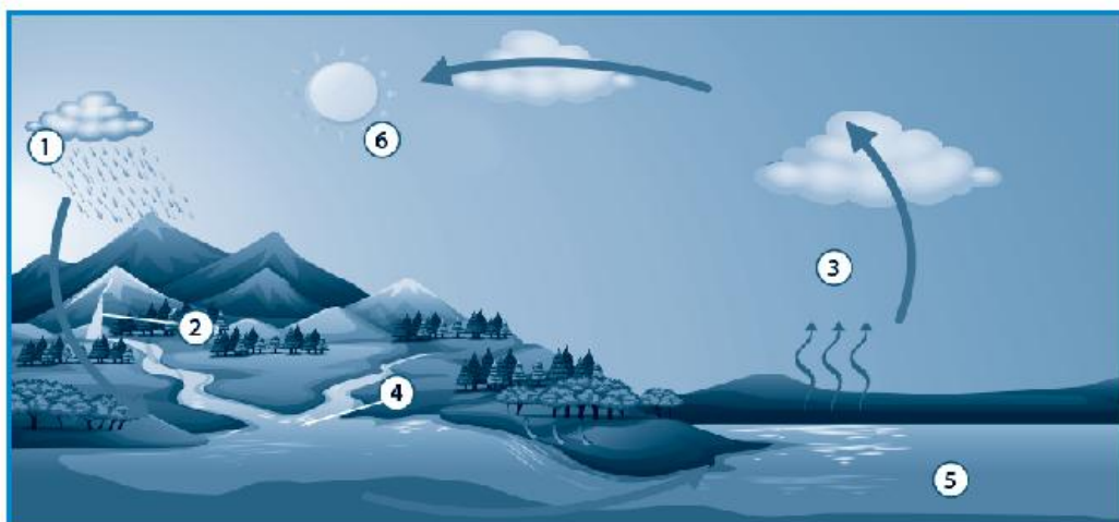
Hình 16.1. Vòng tuần hoàn lớn của nước
