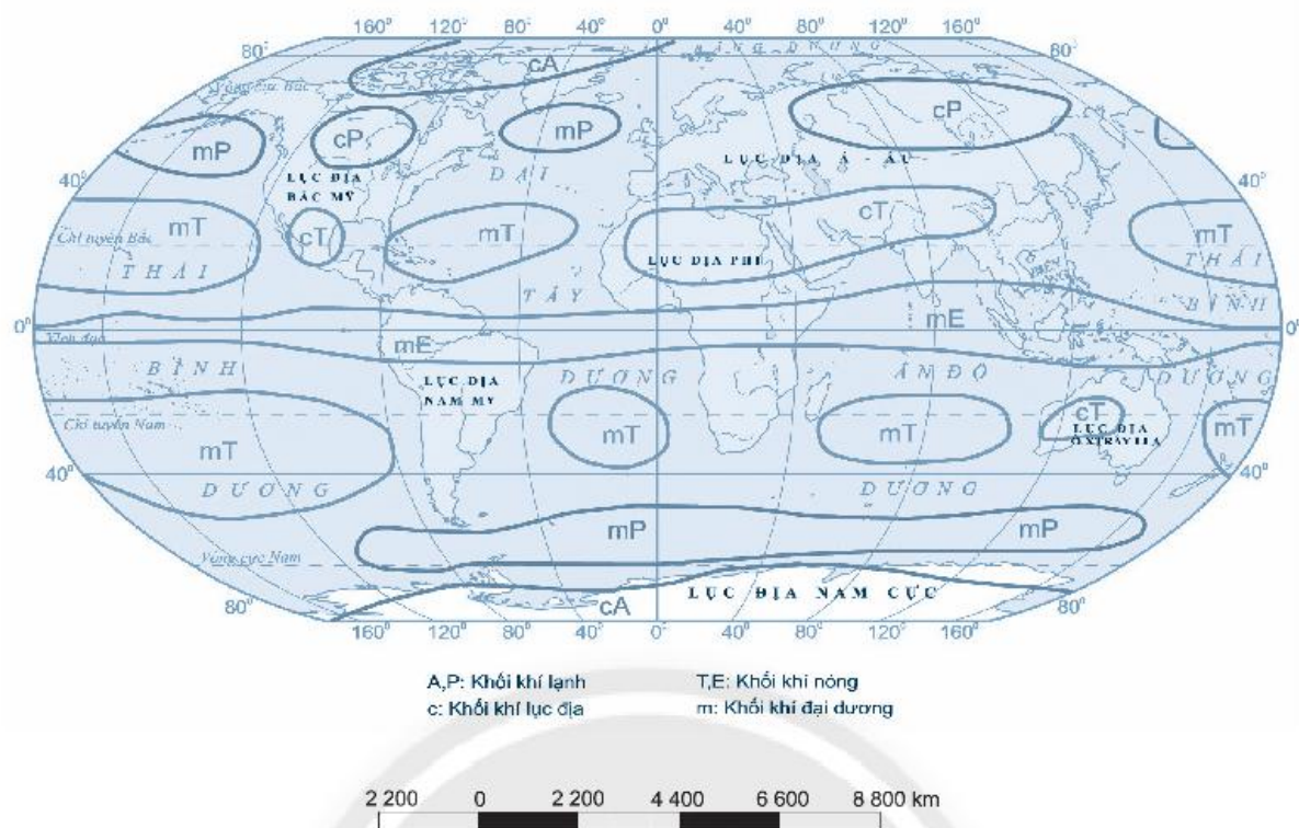
Hình 12.1. Các khối khí trên Trái Đất
