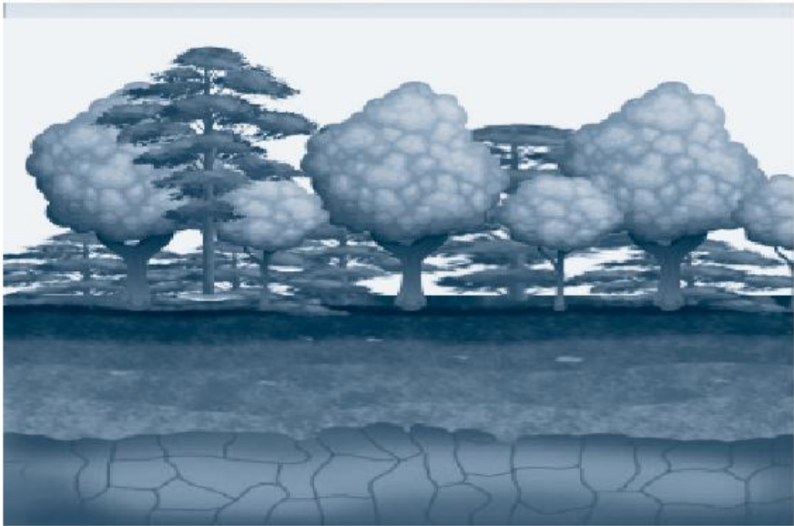
Hình 19.3. Đất ở vùng khí hậu nhiệt đới
