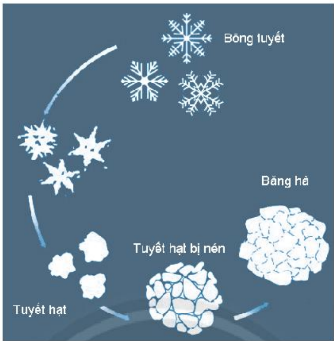
Hình 16.2. Quá trình hình thành băng hà
