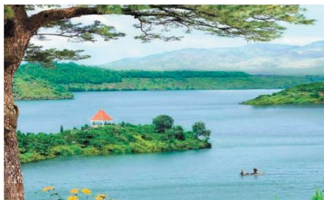
Hình 17.3. Hồ Tơ Nưng (T'Nưng) ở thành phố Pleây-ku (Pleiku), Gia Lai (Việt Nam) được hình thành từ miệng núi lửa đã tắt
