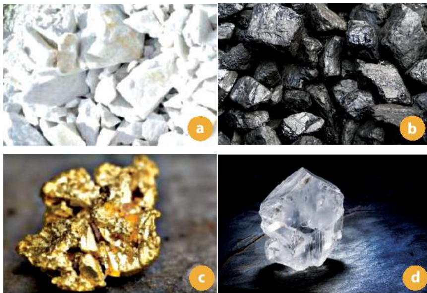
Hình 10.5. Một số loại khoáng sản
