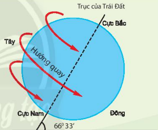
Hình 6.1. Hướng tự quay của Trái Đất
