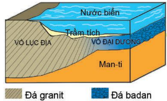
Hình 9.2. Cấu tạo lớp vỏ Trái Đất
