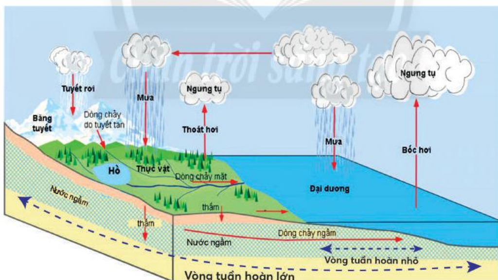
Hình 16.3. Vòng tuần hoàn nước
