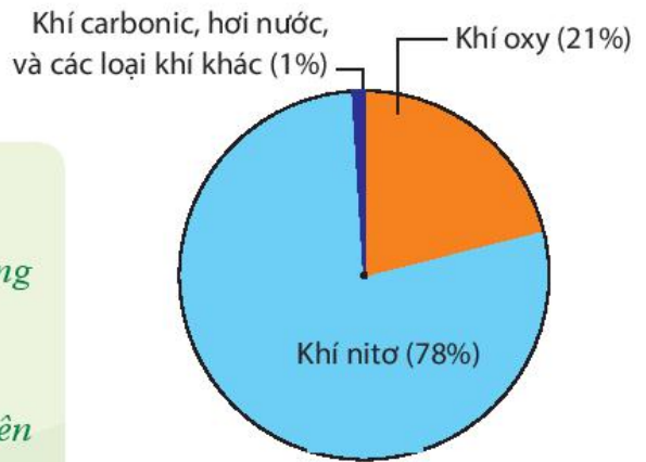
Hình 12.2. Các thành phần của không khí
