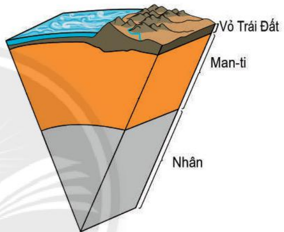
Hình 9.1. Cấu tạo của Trái Đất
