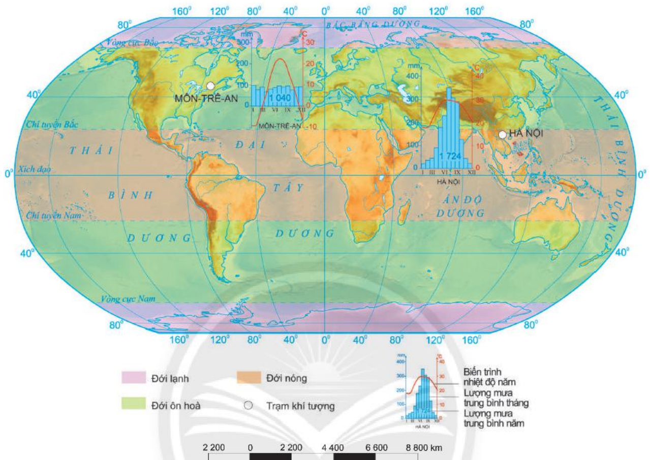
Hình 15.2. Các đới khí hậu trên Trái Đất
