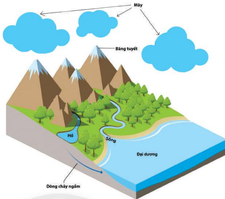
Hình 16.2. Nước trên Trái Đất
