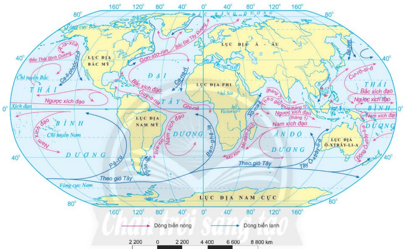
Hình 18.4. Dòng biển trong các đại dương
