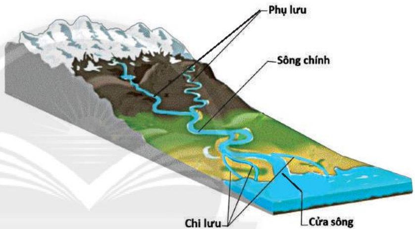
Hình 17.1. Mô hình một hệ thống sông
