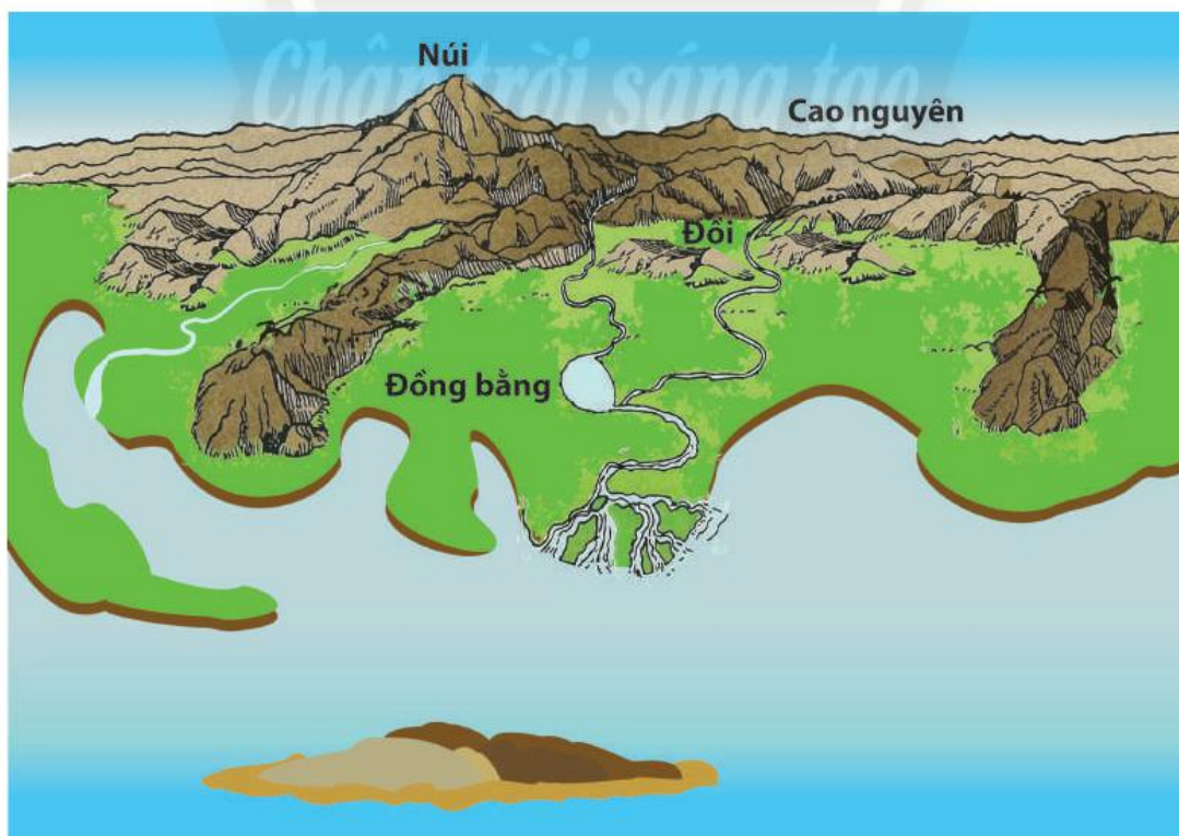
Hình 10.2. Một số dạng địa hình chính
