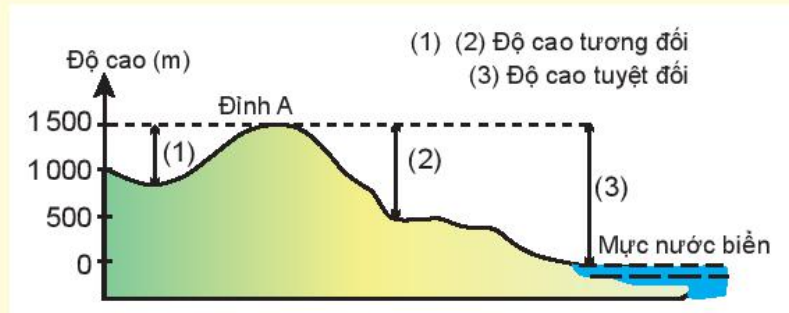
Hình 10.3. Cách tính độ cao địa hình
