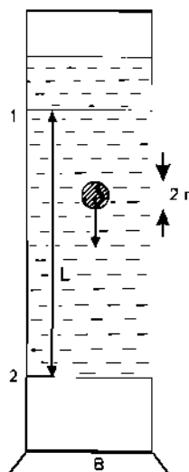
Nhớt kế Nhớt kế bi độ nhớt \eta đo bằng công thức \eta = \frac{mg}{6\pi rL} m - Khối lượng viên bi kim loại có bán kính r; g - Gia tốc trọng trường; t - Thời gian viên bi rơi đều giữa mức 1 và 2 có khoảng cách L trong chất lỏng nhớt trong bình B
