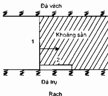
1. Gương lò; 2. Rạch, → hướng chuyển dịch gương lò
