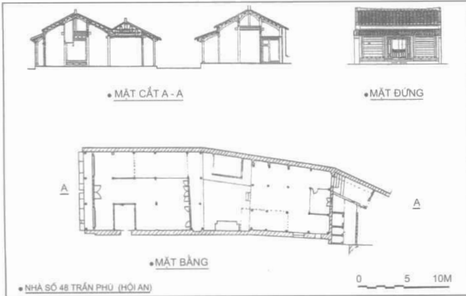
Nhà ống Sơ đồ nhà ống ở Hội An
