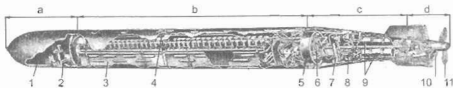
Ngư lôi a) Ngăn thuốc nổ; b) Ngăn ác quy; c) Bộ phận điều khiển; d) Đuôi. 1. Chất nổ; 2. Ngòi nổ; 3. Ác quy; 4. Khí tải đốt hydro; 5. Động cơ điện; 6. Công tắc phồng; 7. Khí tải thủy tinh; 8. Khí tải con quay; 9. Ngăn khí nén; 10. Chân vịt trước; 11. Chân vịt
