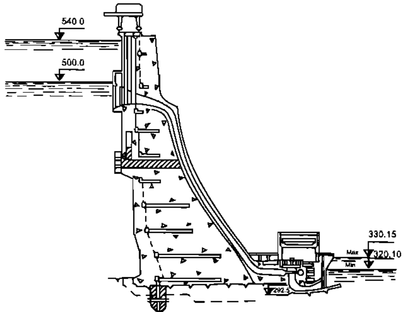
Nhà máy thủy điện sau đập So đồ mặt cắt dọc Nhà máy Thủy điện Xaianô-Susenxkaia
