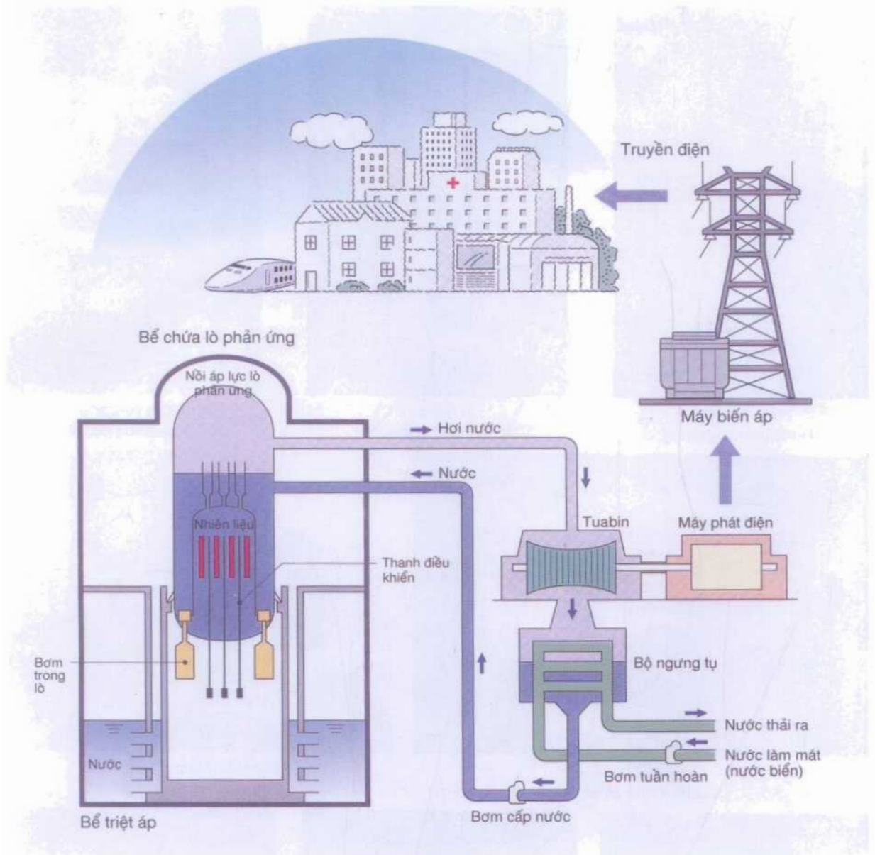
Sơ đồ nguyên lý vận hành nhà máy điện nguyên tử lò nước sôi
