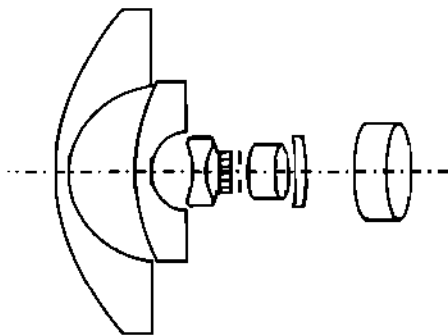
Ống kính mắt cá
