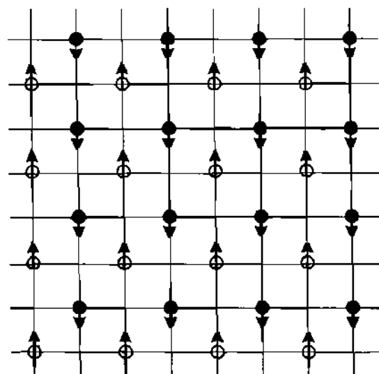
Phản sắt từ Mômen từ của 2 mạng con A và B triệt tiêu nhau ↓ Nguyên tử của mạng con A, ↑ Nguyên tử của mạng con B
