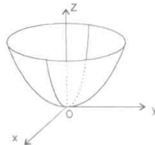
a. Parabôlôit elliptic
