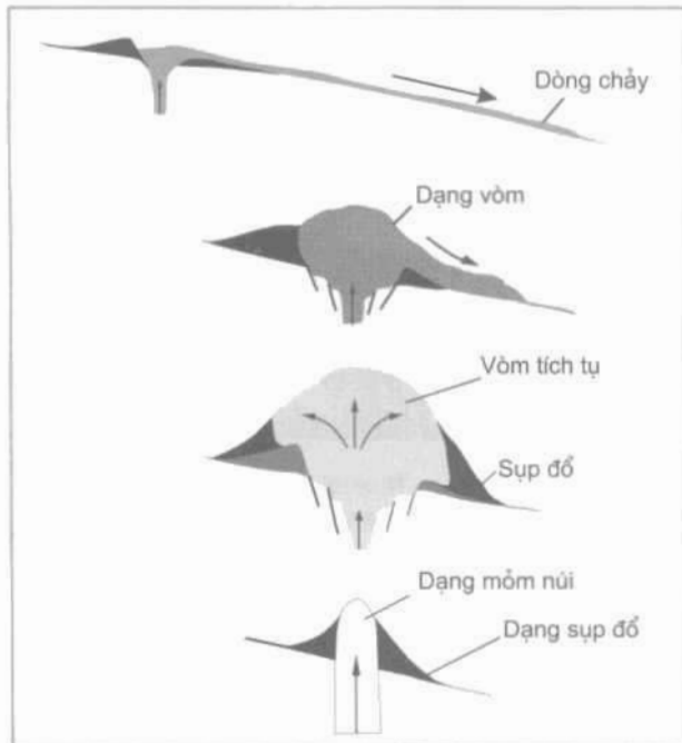
Các dạng núi lửa (theo hình thái)
