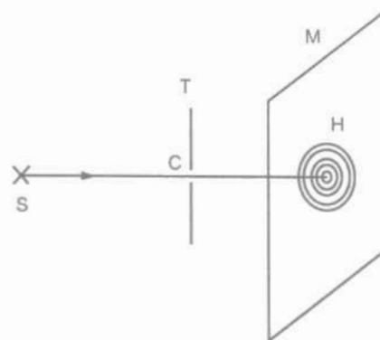
Nhiều xạ ánh sáng
