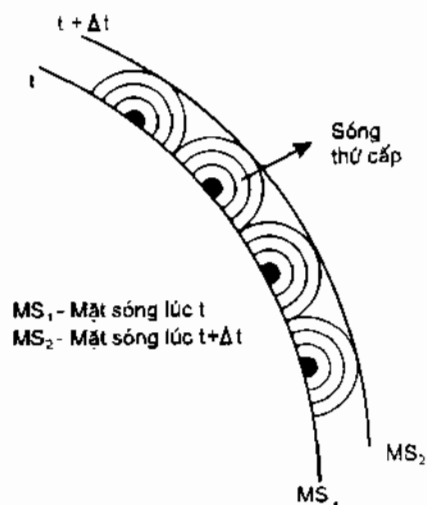
Nguyên lý Huyghen-Frenen
