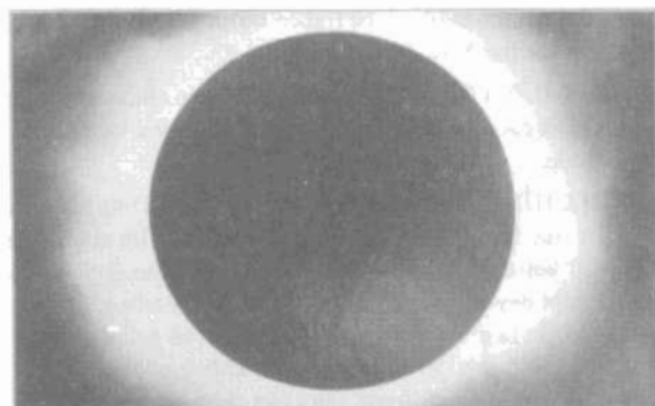
Nhật thực và nguyệt thực Nhật thực toàn phần
