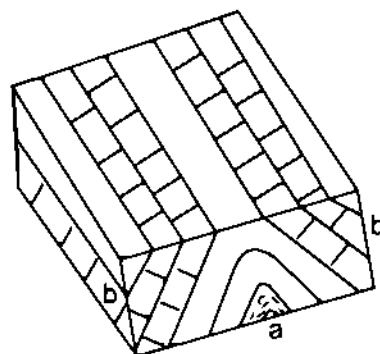
Sơ đồ nếp vồng
