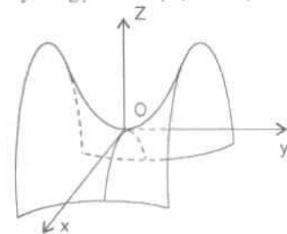
b. Parabôlôit hyperbolic
