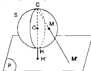
Phép chiếu nổi
