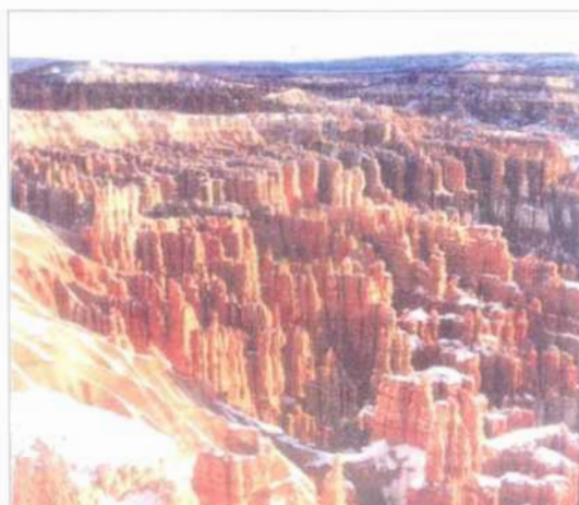
Dạng phong hoá trong hẻm vực
