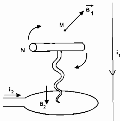
Quy tắc vận nút chai
