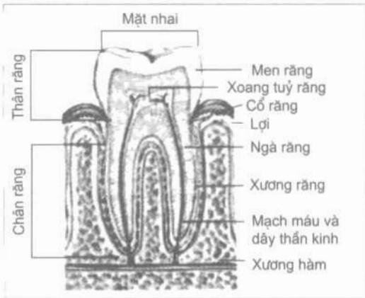
Răng Mặt cắt dọc một chiếc răng người
