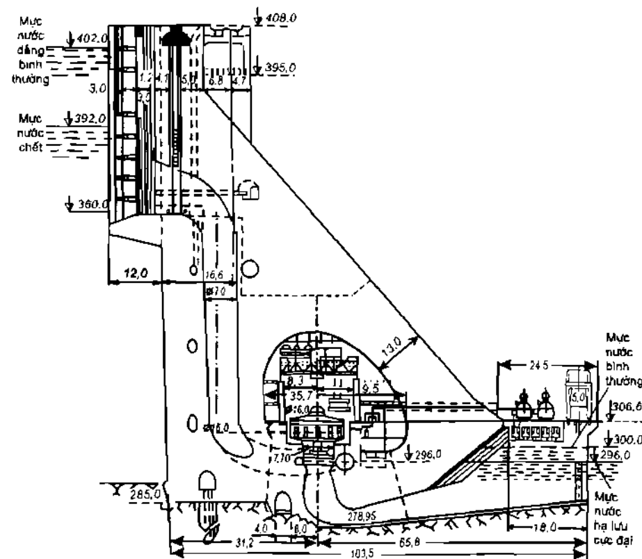
Nhà máy thủy điện trong thân đập Sơ đồ mặt cắt dọc nhà máy thủy điện trong thân đập
