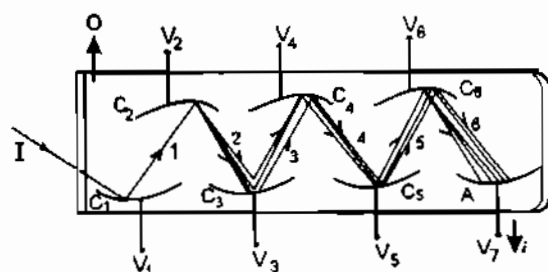
Ống nhân quang điện
