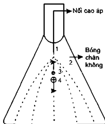
Nguồn ion trong kính hiển vi ion
