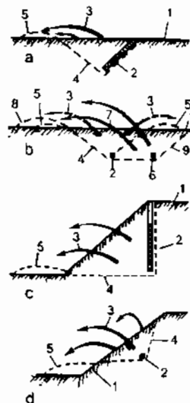
Nổ mìn định hướng
