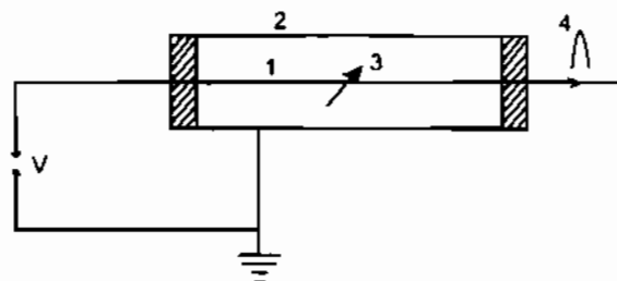
Ống đếm Gaigơ
