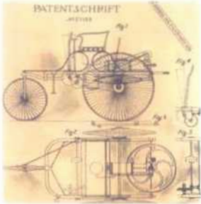
Bằng sáng chế ô tô cấp cho K. Benxơ ngày 2.11.1886
