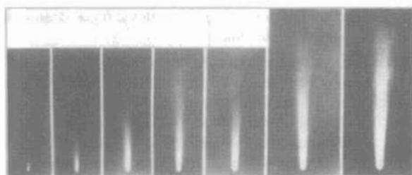
Sao chổi Halây
