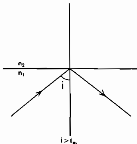
Phản xạ nội toàn phần
