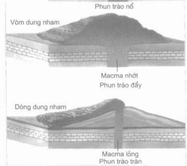
Phun trào Các dạng phun trào chính
