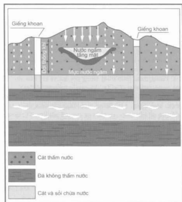
Nước dưới đất Mặt cắt dọc của nước dưới đất
