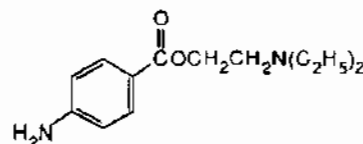
Novocain
