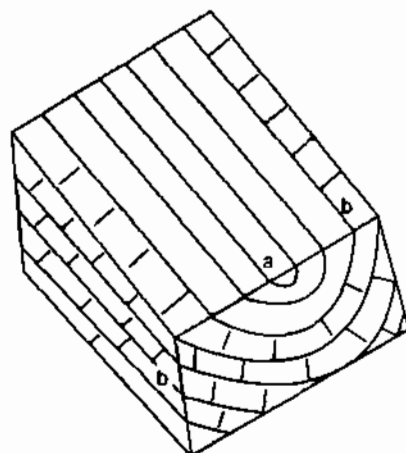
Sơ đồ nếp lõm
