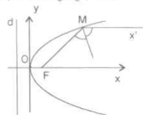
Parabôn
