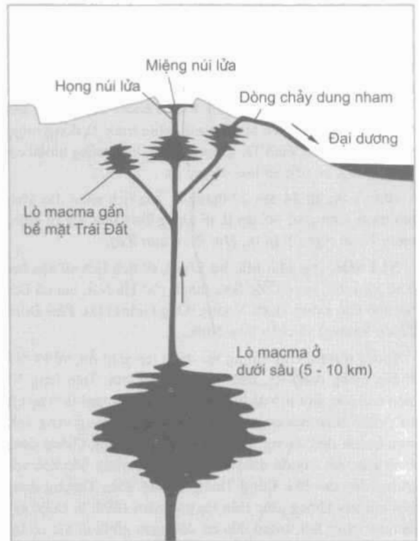
Cơ cấu núi lửa (Chỏm núi Funezơ)
