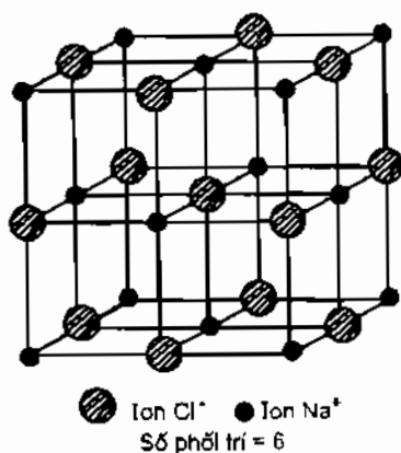
Số phối trí
