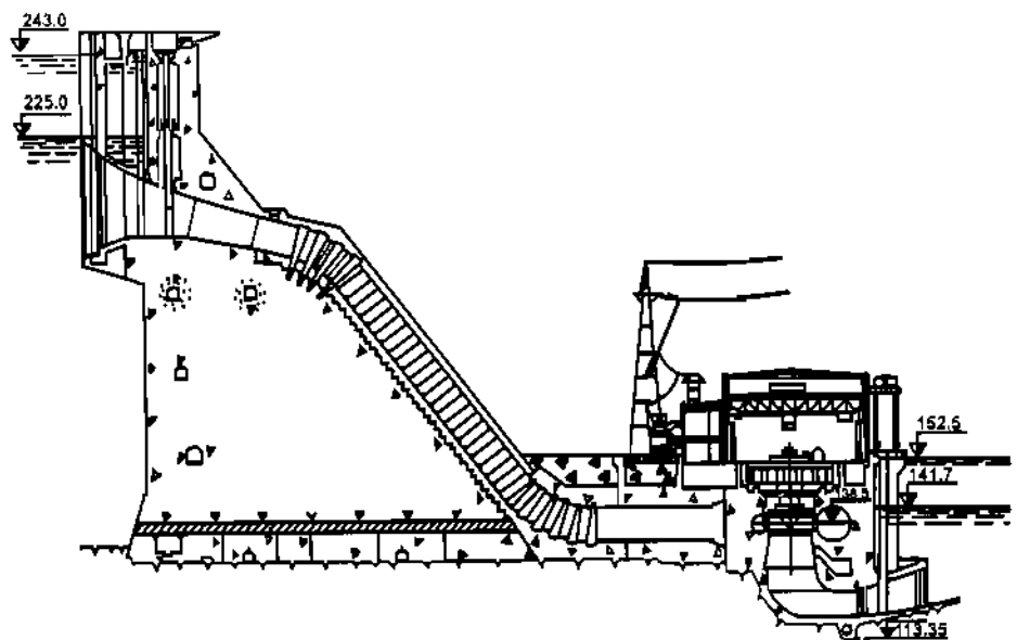
Nhà máy thủy điện sau đập So đồ mặt cắt dọc Nhà máy Thủy điện Krasnojarsk
