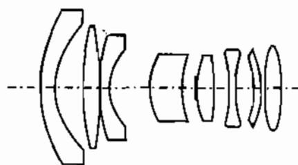
Ống kính góc rộng tiêu điểm lùi
