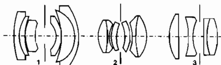
Ba loại ống kính hiện đại: 1. Ống kính góc rộng không tiêu điểm lùi, 2. Ống kính loại Gauss (Gauss) kép, 3. Ống kính đối xứng gồm bốn thấu kính. Ống kính góc rộng
