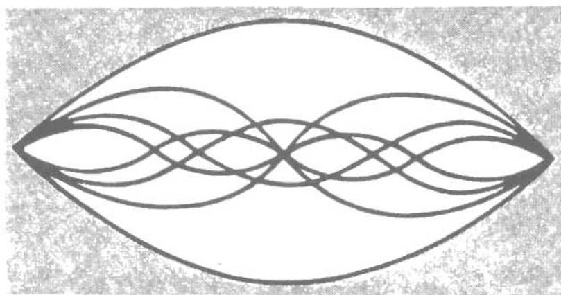
Biểu đồ này minh họa một dây đàn dao động từng phần và toàn phần. Dao động dài nhất xác định cường độ, còn những dao động nhỏ hơn tạo ra sự hòa âm.
