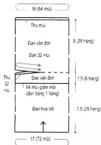
Cách đan gót sau
