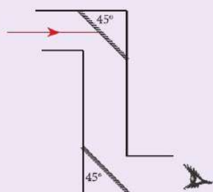
Hình 13.8. Sơ đồ kính tiềm vọng đơn giản
