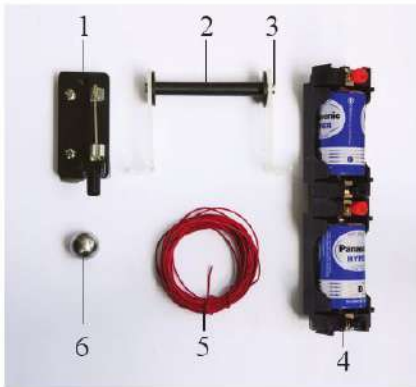
Hình 15.7. Bộ dụng cụ chế tạo nam châm điện
