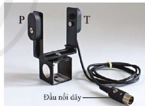
Hình 4. Cổng quang điện
