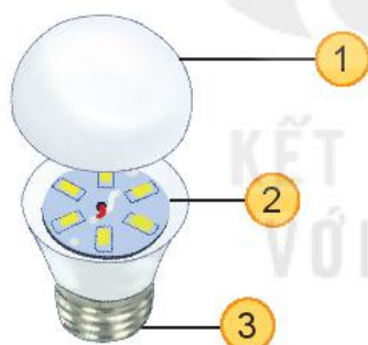
Hình 11.5. Cấu tạo của bóng đèn LED búp
