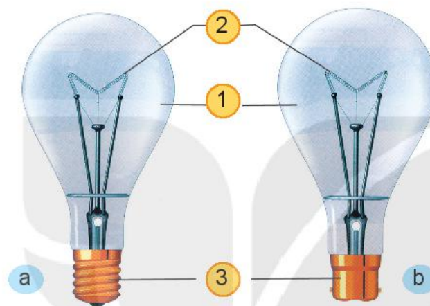
Hình 11.2. Cấu tạo của bóng đèn sợi đốt
