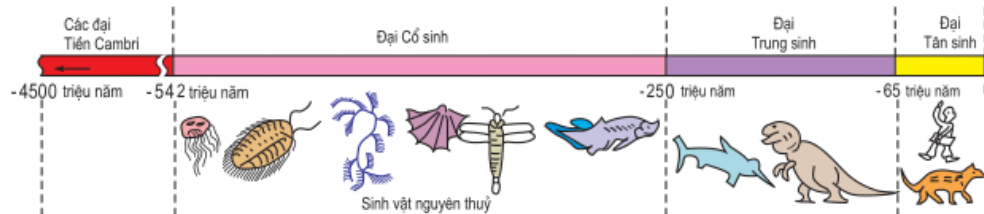
Bảng 25.1. Niên biểu địa chất (rút gọn)
