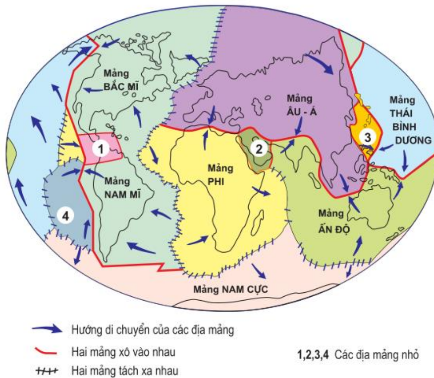
Hình 19.2. Lược đồ các mảng kiến tạo
