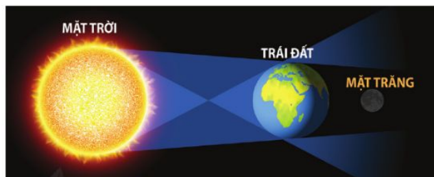
Hiện tượng Nguyệt thực
