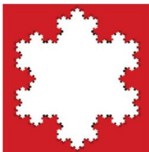
Bông tuyết Koch (Minh họa: Astronira)
