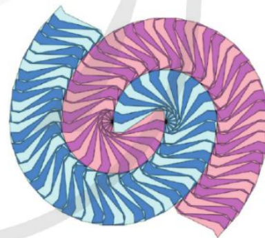
Xoắn đơn của Heinz Voderberg
