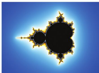
Fractal Mandelbrot (Minh họa: Vit Smolek)
