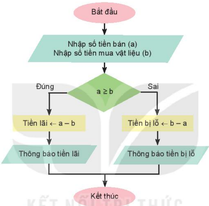
Hình 6.14. Sơ đồ khối mô tả thuật toán tính toán tiền bán thiệp chúc mừng
