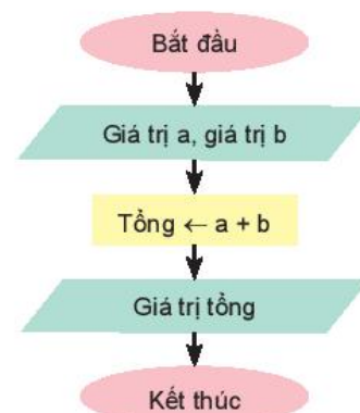
Hình 6.3. Sơ đồ khối
