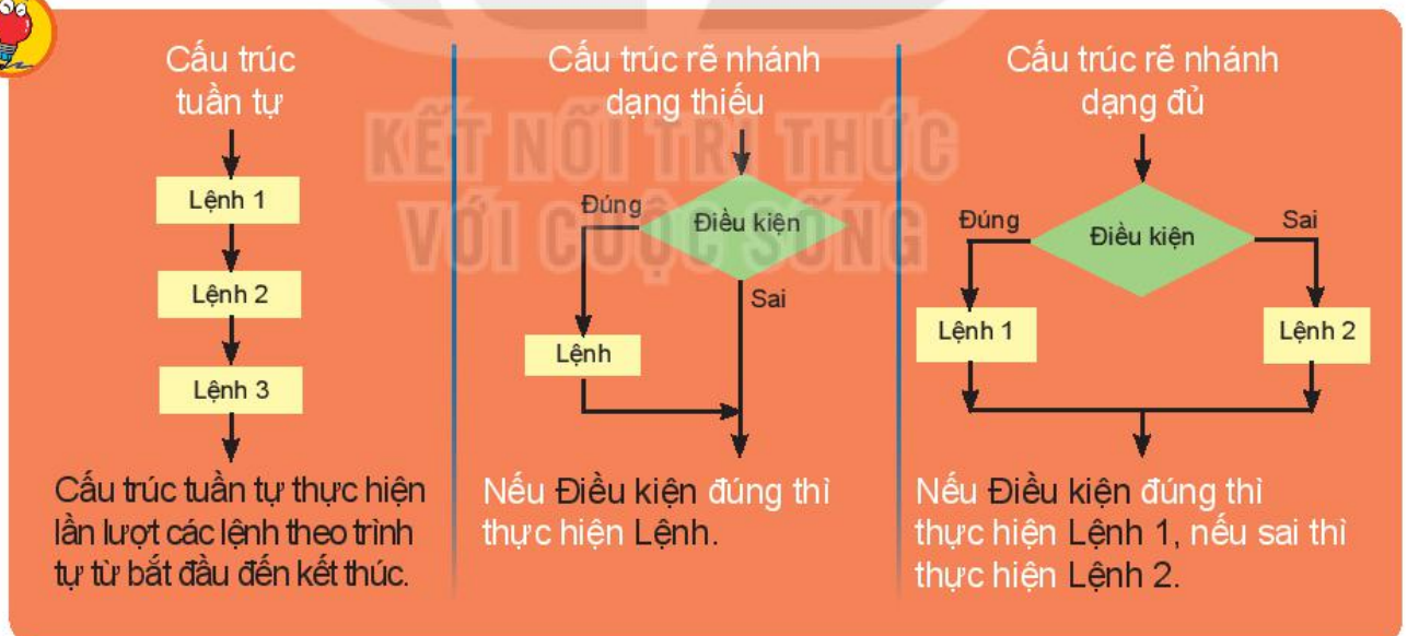
Hình 6.8. Sơ đồ khối mô tả cấu trúc rẽ nhánh dạng đủ
