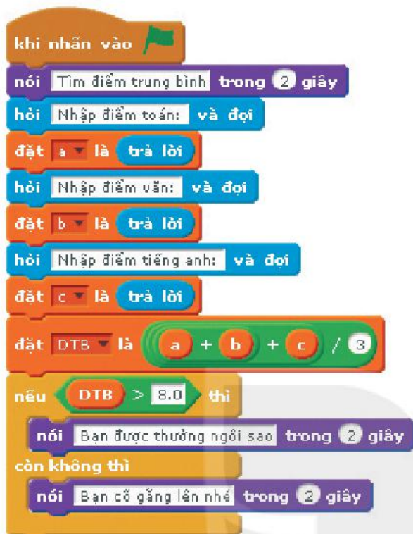
Hình 6.15. Chương trình Scratch
