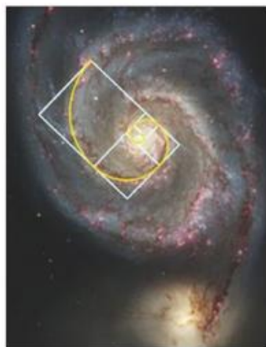
Dải ngân hà NGC 5 194
