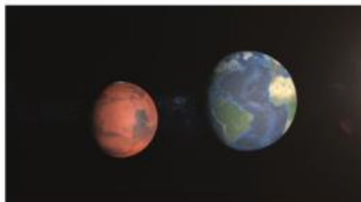
Hình ảnh Sao Hỏa và Trái Đất
