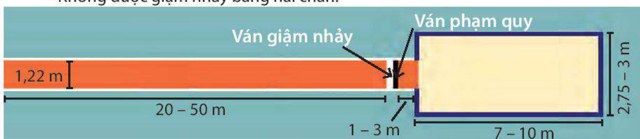
Hình 3. Kích thước sân nhảy xa
