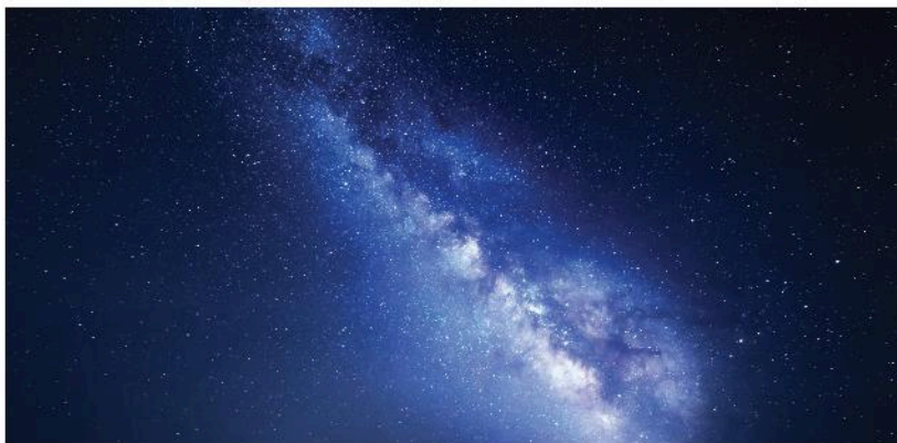
▲ Hình 45.5. Dải Ngân Hà quan sát từ Trái Đất
