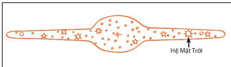
▲ Hình 45.7. Mô hình phác hoạ Ngân Hà và vị trí Mặt Trời trong hệ Ngân Hà
