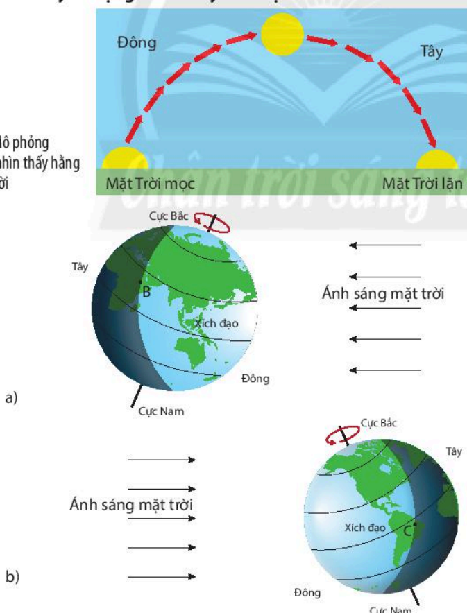
▲ Hình 43.2. Mô phỏng chuyển động tự quay quanh trục của Trái Đất
