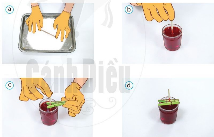
Hình 10.8. Thí nghiệm về quá trình kết tinh đường ăn
