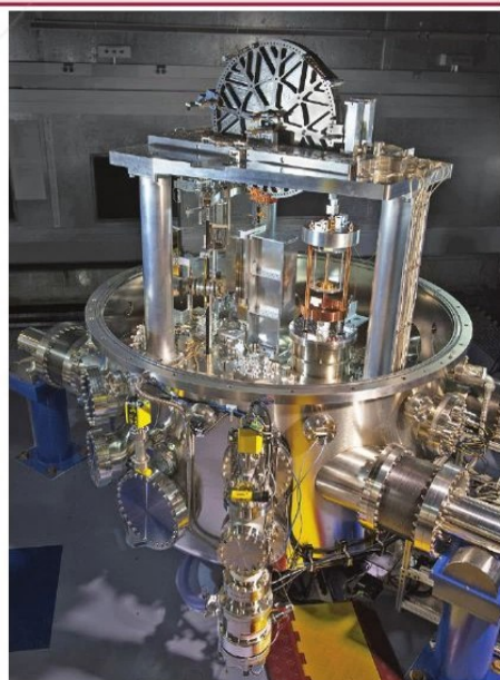
Hình 3.7. Cân Kíp-bơ
