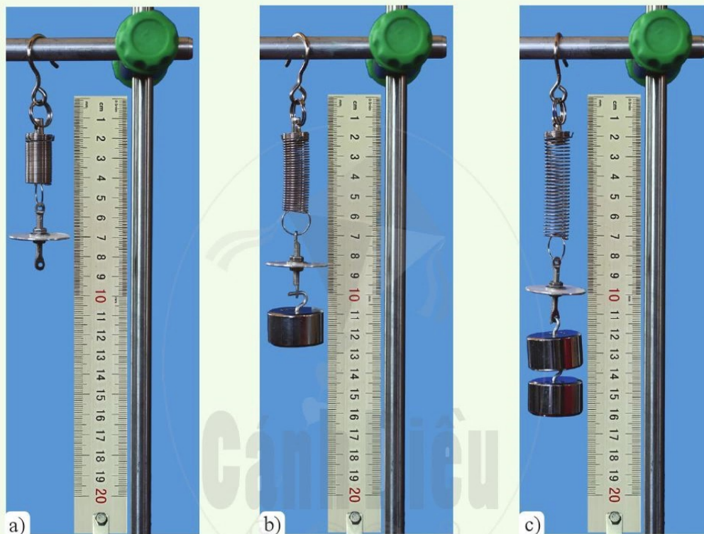
Hình 29.3. Thí nghiệm về độ giãn của lò xo
