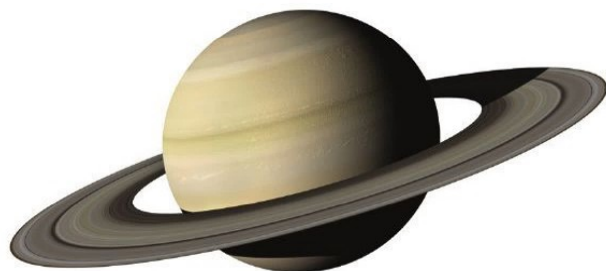
Hình 35.4. Thổ Tinh
