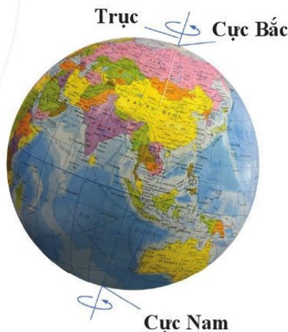
Hình 33.1. Trái Đất quay quanh trục
