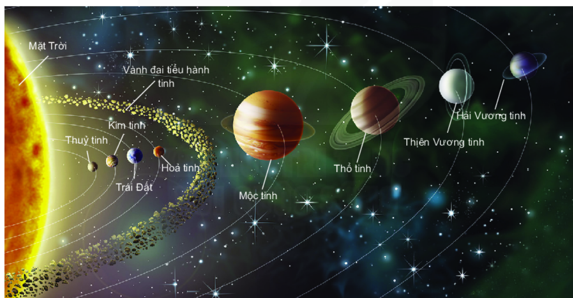
Hình 3.1 Các hành tinh của Hệ Mặt Trời tính từ trong ra ngoài: Thủy tinh, Kim tinh, Trái Đất, Hỏa tinh, Mộc tinh, Thổ tinh, Thiên Vương tinh, Hải Vương tinh.
