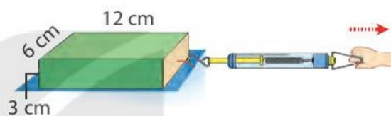
a) Đo lực ma sát trượt của miếng gỗ có diện tích tiếp xúc là 12 cm x 6 cm
