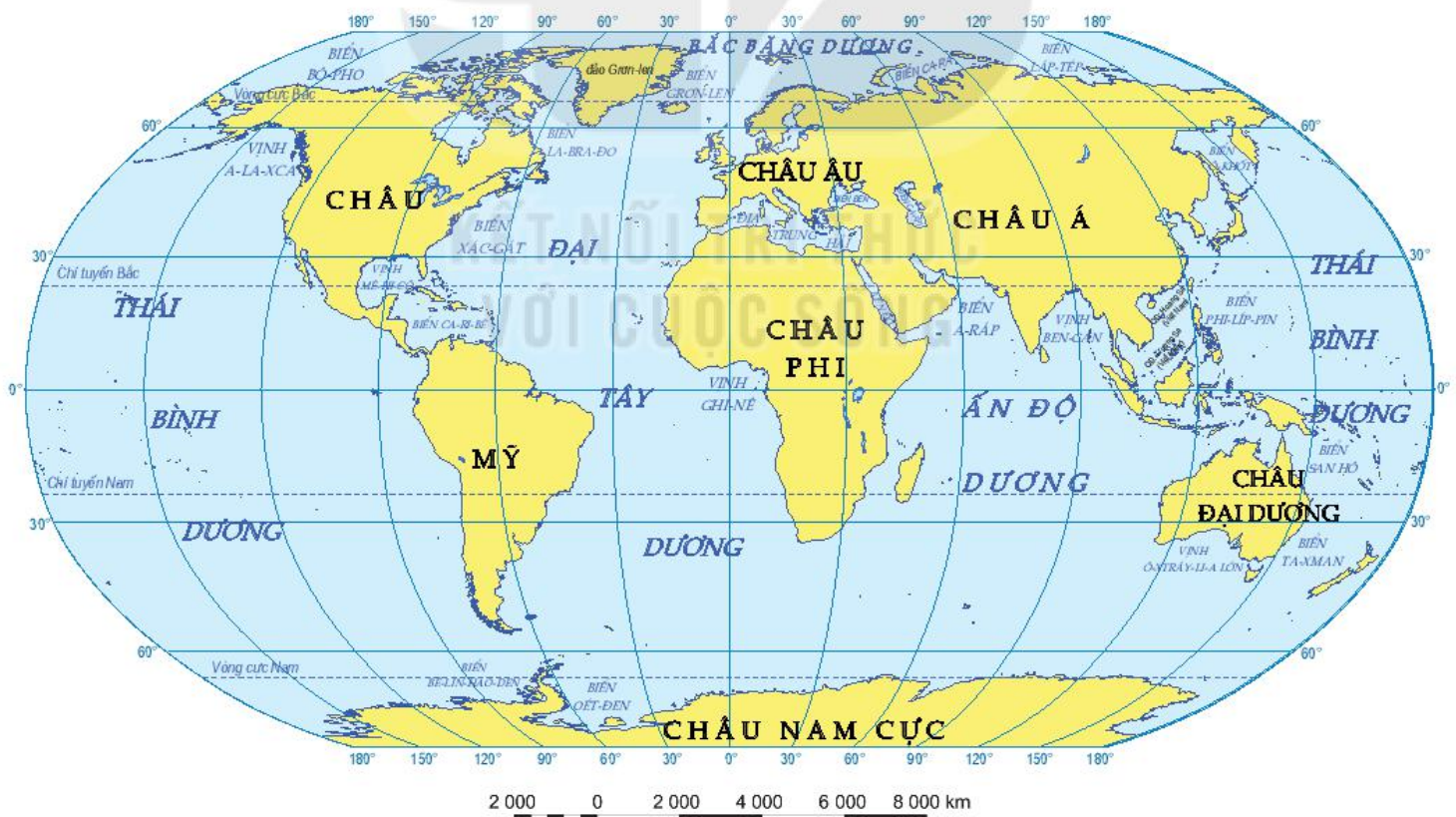
Hình 1. Biểu và đại dương trên thế giới
