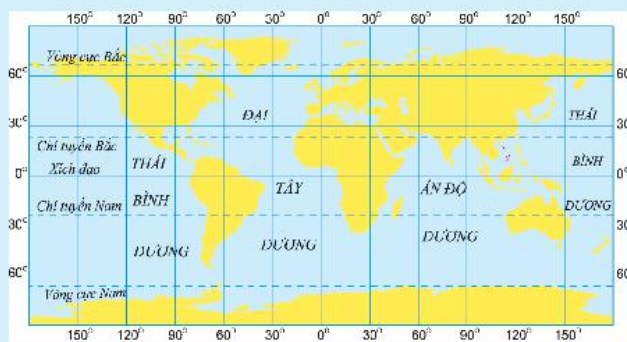
b) Lưới kinh, vĩ tuyến của phép chiếu hình trụ
