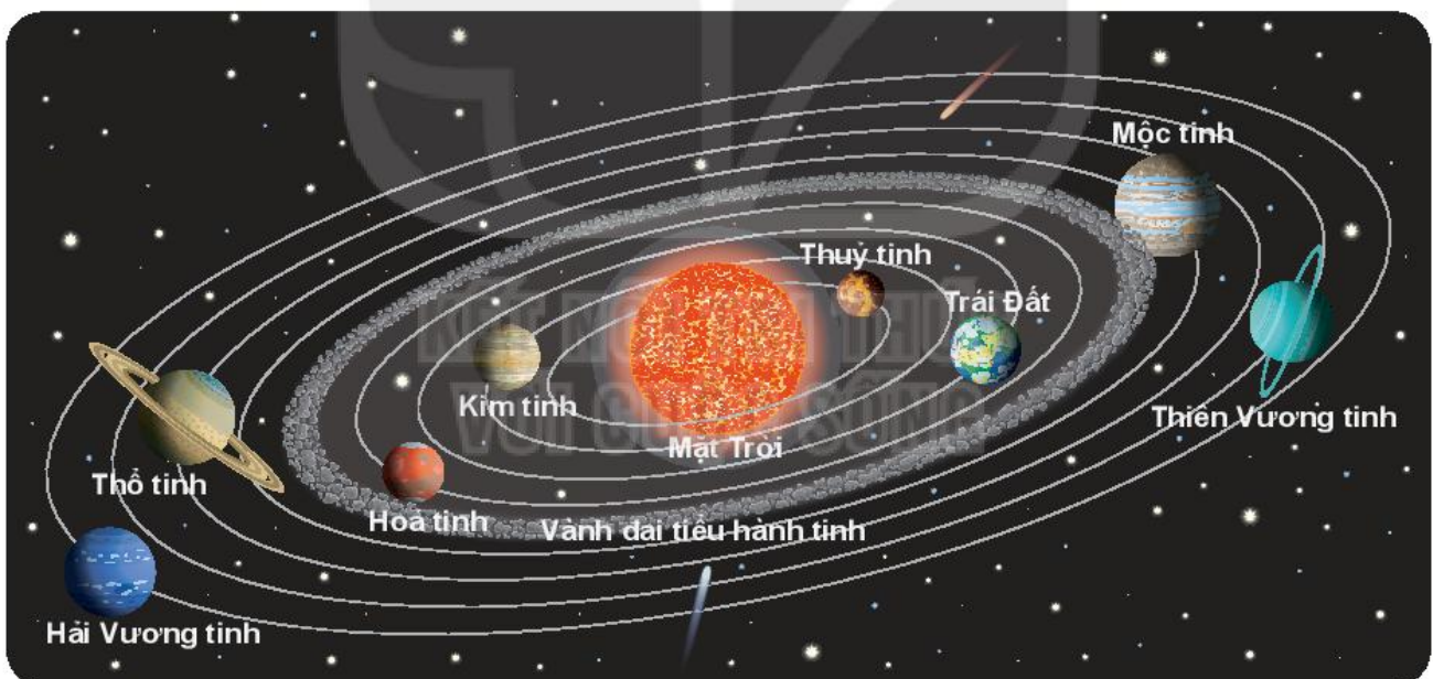
Hình 1. Các hành tinh trong hệ Mặt Trời
