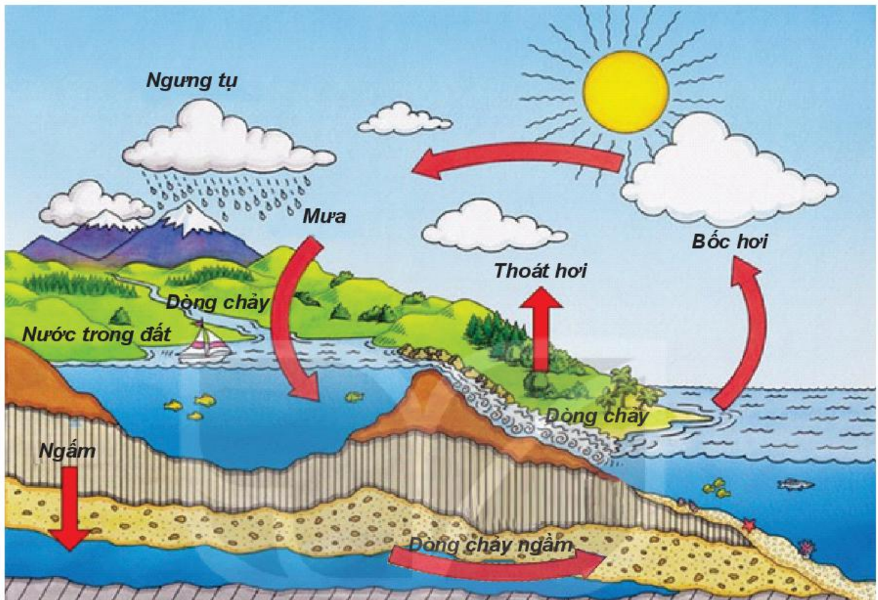
Hình 2. Vòng tuần hoàn lớn của nước
